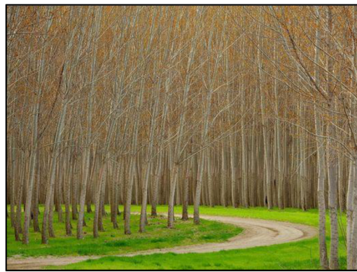
Obr. 5.1 Japonský topol [28]
