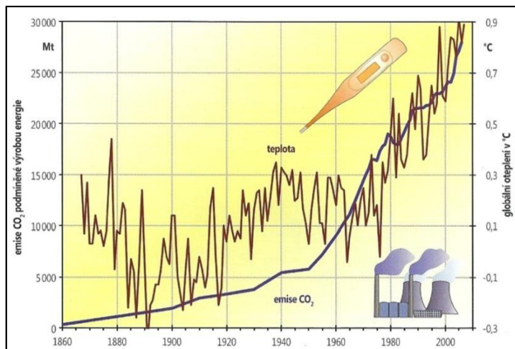
Obr. 1.2 Vývoj emisí CO 2 a globální změny teploty [1]
