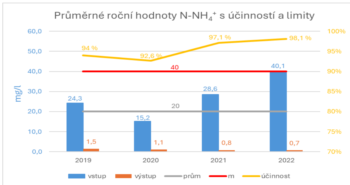
Obrázek 19 - Průměrné roční hodnoty N-NH 4 + v letech 2019 – 2022 na vstupu a výstupu z BČOV se stanovenými limity a účinností čistírny
