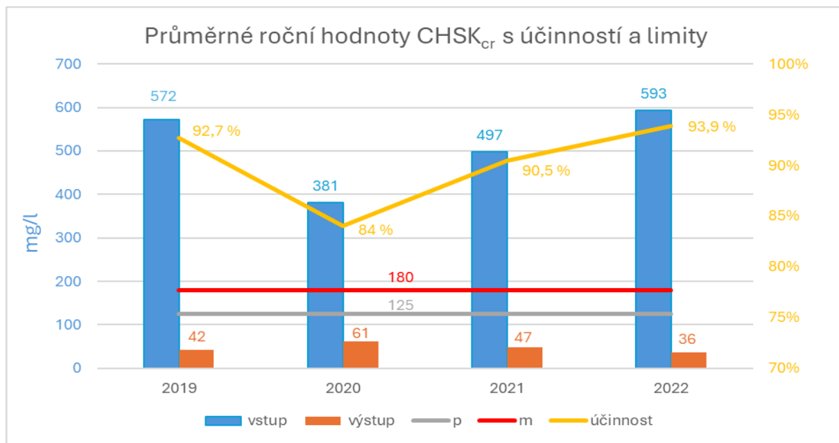
Obrázek 15 - Průměrné roční hodnoty CHSK Cr v letech 2019 – 2022 na vstupu a výstupu z BČOV se stanovenými limity a účinnostmi čistírny
