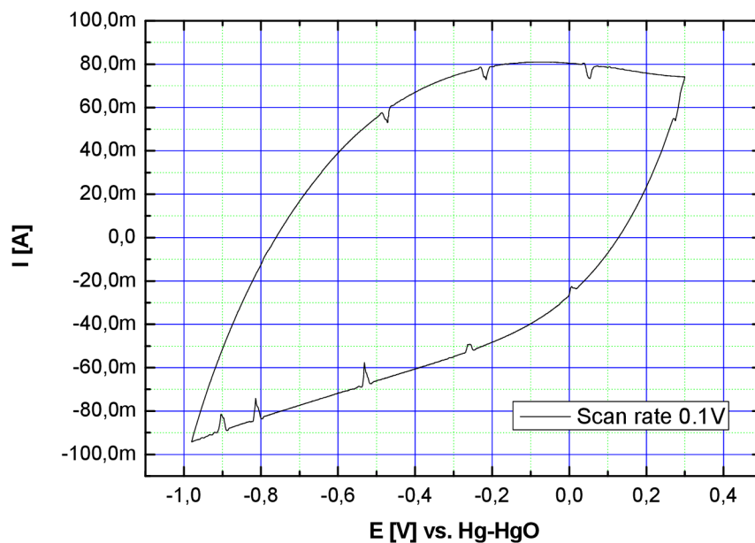
Obr. 9.18: CV na síťkové elektrodě – elektroda č. 2, 1cm 2 , Chezacarb A + 30 hm. % Raneyova Ni – v 1M KOH, bubláno H 2 , scan rate 0,1V
