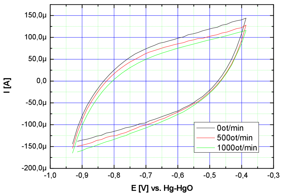
Obr. 9.11: CV na RDE – Chezcarb A + Pt – v 1M KOH, vodík, scan rate 0,01V při 0, 500 a 1000 ot. / min
