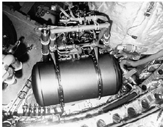
Obr. 2.5: Palivový článek (PEM) pro vesmírný program Gemini (1963) [5]
