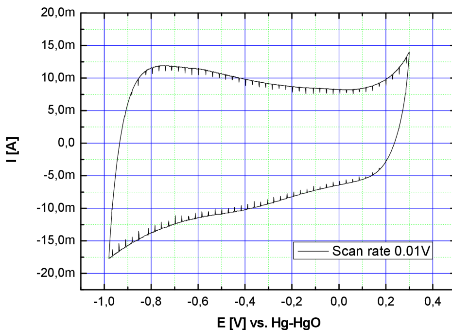
Obr. 9.19: CV na síťkové elektrodě – elektroda č. 2, 1cm 2 , Chezacarb A + 30 hm.% Raneyova Ni – v 1M KOH, bubláno H 2 , scan rate 0,01V
