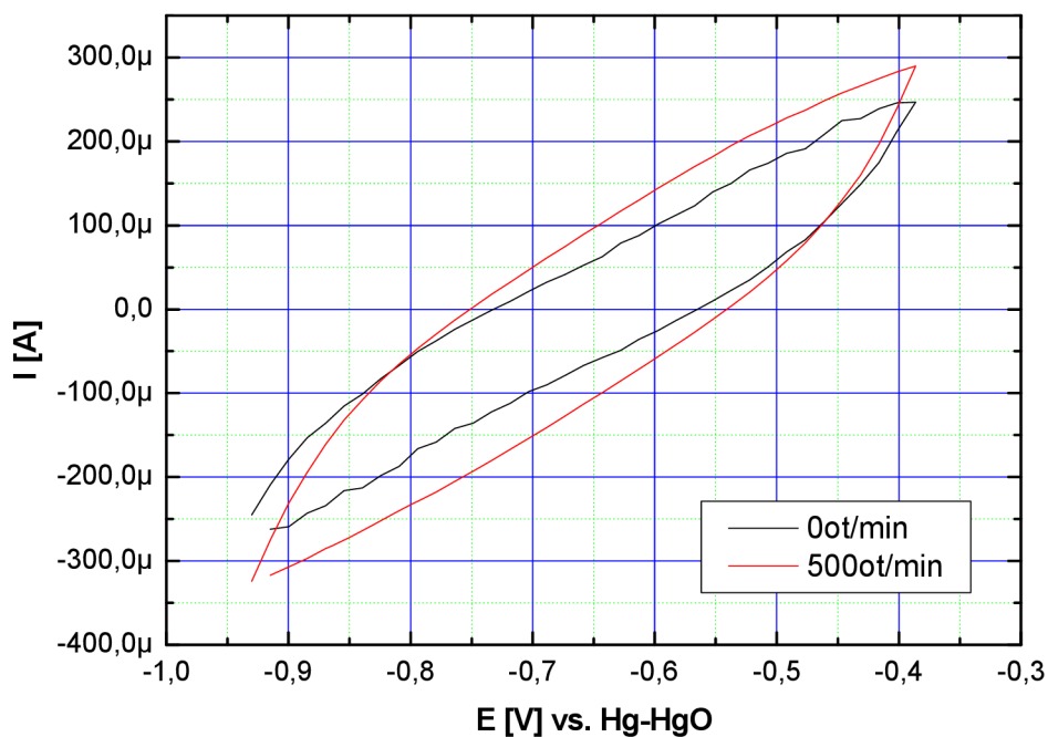
Obr. 9.23: CV na RDE – Chezacarb A + Raney Ni – v 1M KOH + dusík, scan rate 0,1V při 0 a 500 ot. / min
