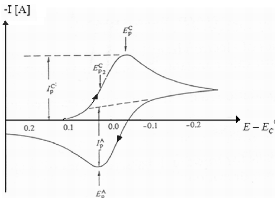
Obr. 6.6: Typický průběh polarizační křivky při cyklické voltametrii (CV) [7]
