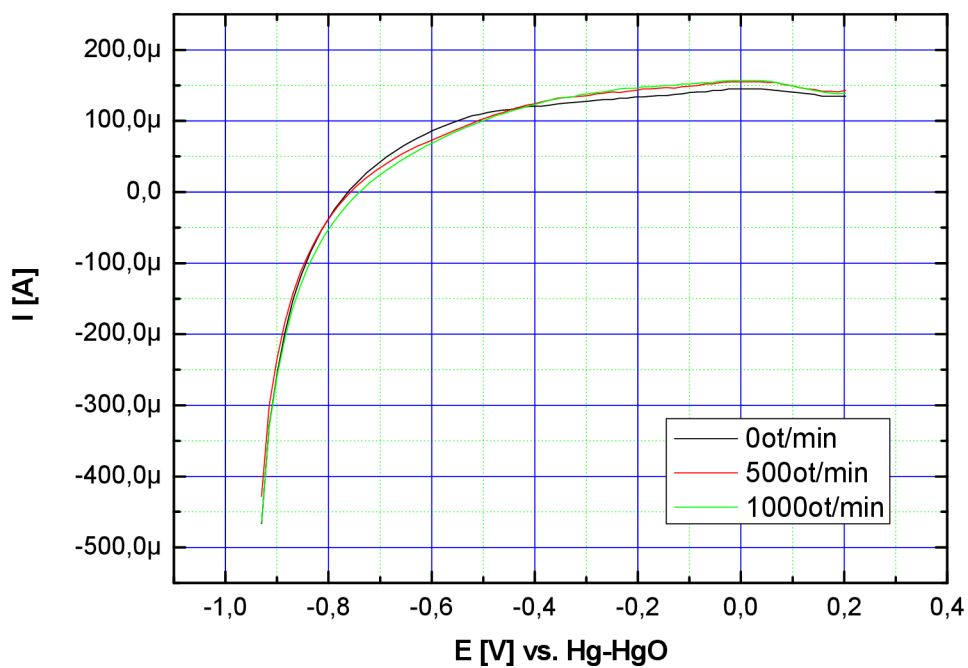
Obr. 9.12: LSV (linear sweep voltametry) - Hydrodynamika na RDE – Chezcarb A + Pt – v 1M KOH, vodík při 0, 500 a 1000 ot. / min
