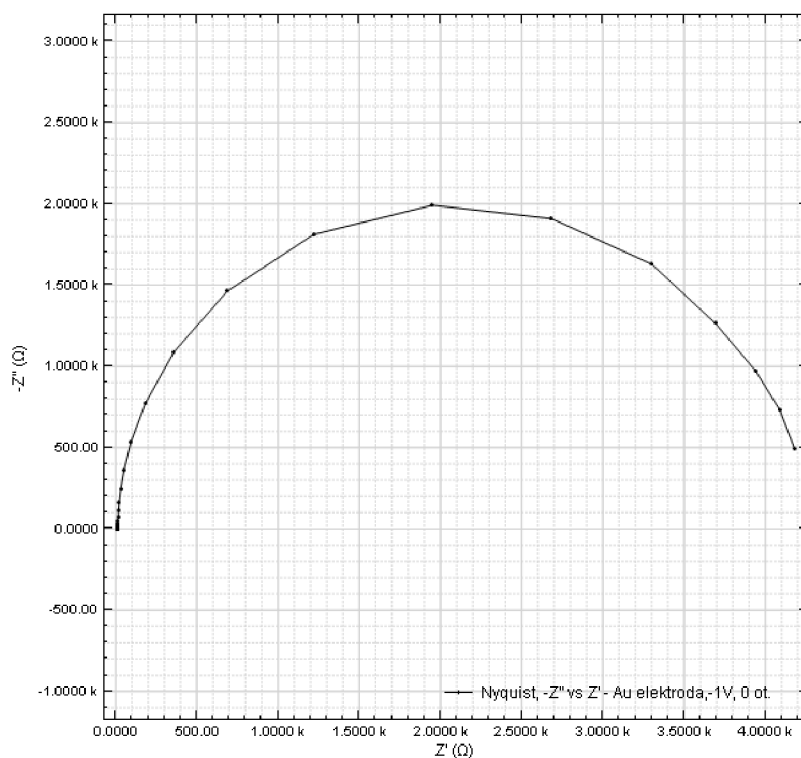
Obr. 6.1: Impedanční spektroskopie – ukázka Nyquistova diagramu
