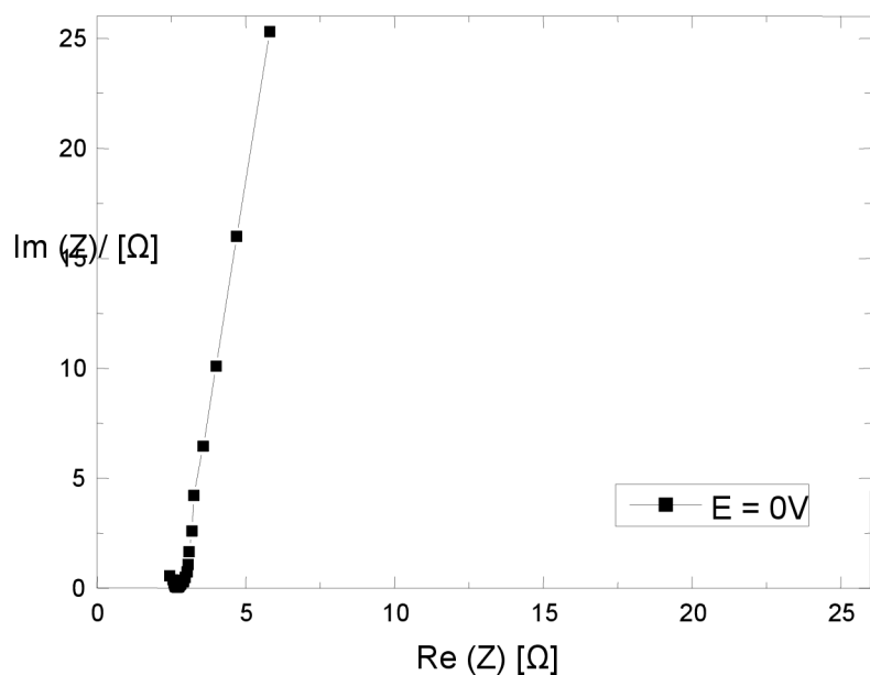
Obr. 9.22: FRA na síťkové elektrodě – elektroda č. 2, 1cm 2 , Chezacarb A + 30 hm. % Raneyova Ni – v 1M KOH, bubláno H 2 , E = 0V vs. Hg – HgO
