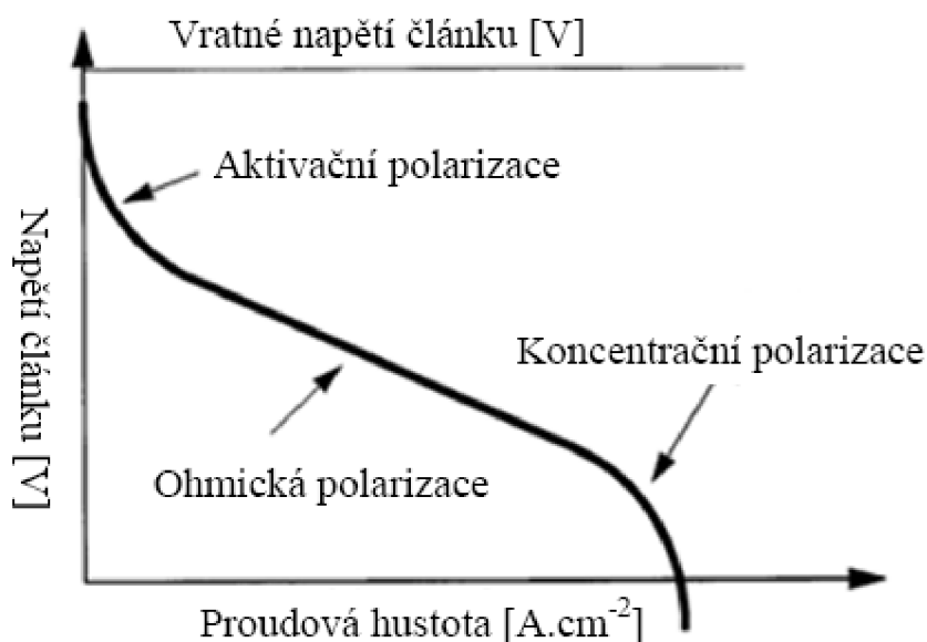
Obr. 4.1: Úbytek napětí PČ při zatížení [1]
