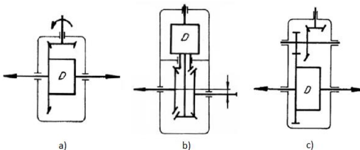
Obr. 3.1 a) jednoduchý stálý převod, b) dvoustranný stálý převod, c) dvojnásobný stálý převod [14]
