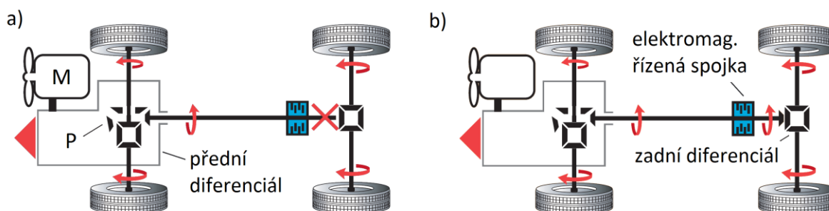
Obr. 6.10 Schéma systému s elektromagneticky ovládanou spojkou v režimu pohonu: a) jedné nápravy, b) všech kol [17]
