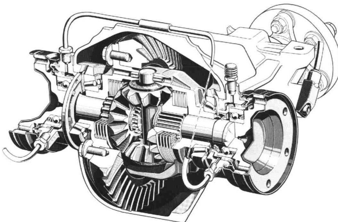
Obr. 3.14 Řez samočinným samosvorným diferenciálem ASD [31]
