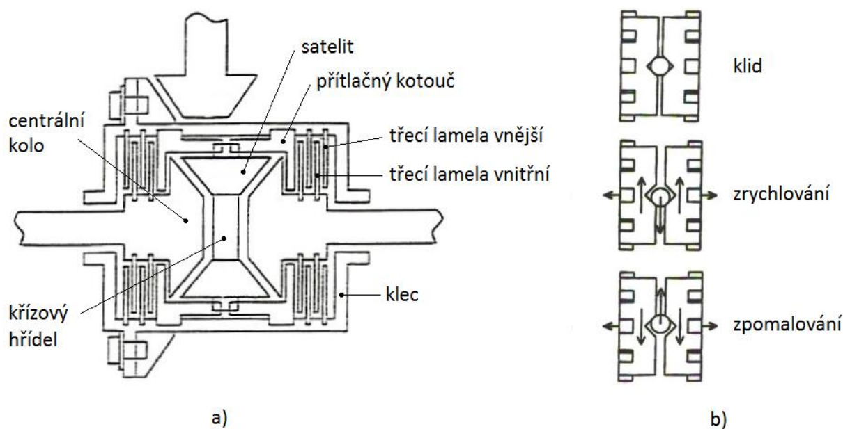
Obr. 3.9 schéma a) SDs třecí lamelovou spojkou, b) mechanismu, vytvářejícího tlak na lamely [21]
