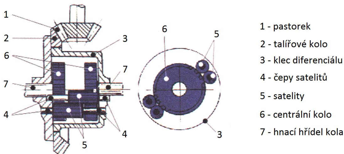
Obr. 3.8 Čelní diferenciál s přímými zuby [13]
