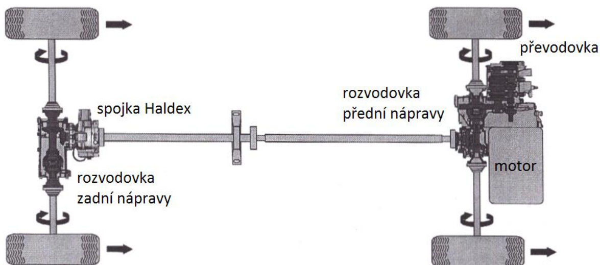
Obr. 6.5 Schéma pohonu vozu Octavia Combi 4x4 2001 [76]
