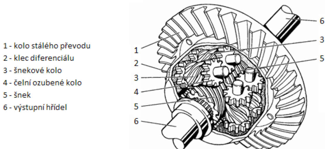
Obr. 3.11 Diferenciál Torsen typ A [26]
