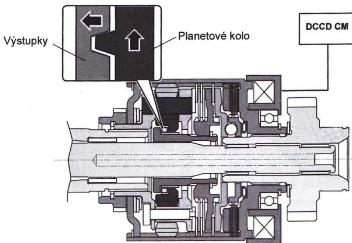
Obr. 6.8 Mezinápravový diferenciál s aktivovaným mechanickým závěrem [1]
