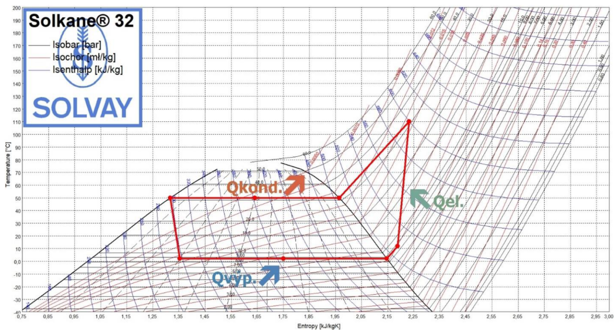
Obr. 25 T-S diagram okruhu TČ
