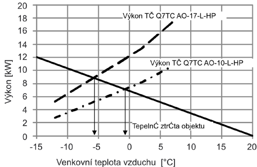
Obr. 19 Závislost výkonu TČ vzduch-voda na venkovní teplotě vzduchu [27]
