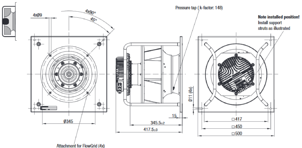
Obr. 26 Ventilátor RadiPac série K3G355 [30]
