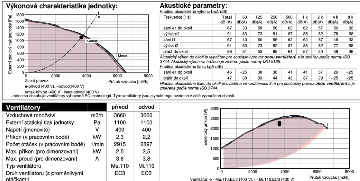
Obr. 43 Hodnoty akustického výkonu jednotky ROTO-N 5000 v pracovním bodě denního režimu
