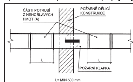
Obr. 45 Prostup vzduchotechnického potrubí s požární klapkou osazenou v požárně dělicí konstrukci [61]
