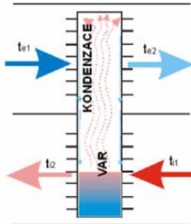
Obr. 4 Schéma zařízení ZZT s tepelnými trubicemi [6]
