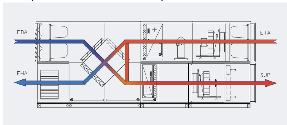
Obr. 12 Schéma uspořádání součástek VZT jednotky dle konfigurace 2 [17]
