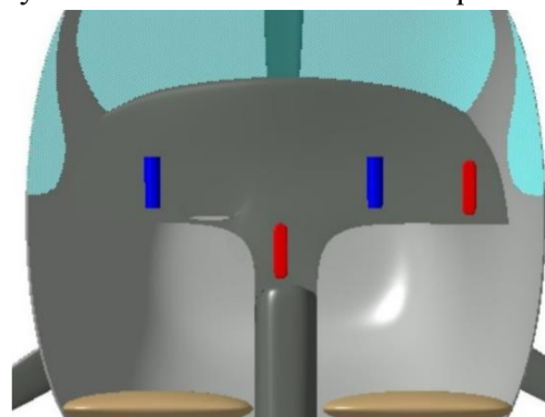
Obr. 25 – Rozmístění řídicích pák na palubní desce
