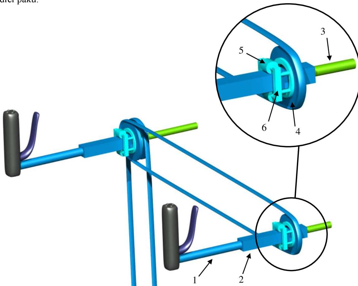
Obr. 28 – Schéma soustavy s dvojitým řízením křidélek: 1) ovládání křidélek, 2) hranolová část ovládání křidélek, 3) ovládání výškového kormidla, 4) ozubené kolo, 5) pojezdový váleček, 6) domek
