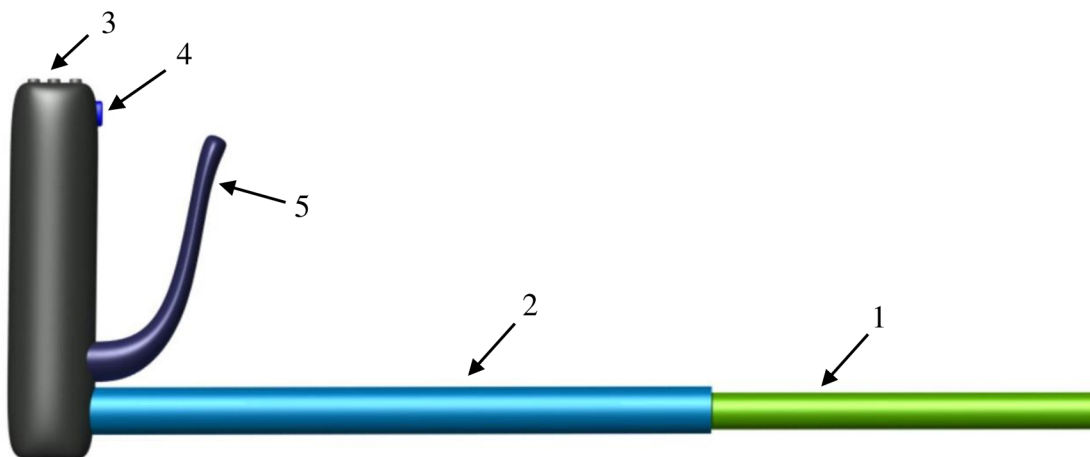
Obr. 26 – Řídicí páka křidélek a výškového kormidla: 1) ovládání výškového kormidla, 2) ovládání křidélek, 3) tlačítka trimu, 4) tlačítko vysílačky, 5) brzda podvozku
