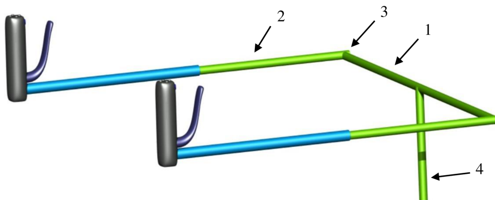
Obr. 27 – Schéma soustavy dvojitého řízení výškového kormidla: 1) propojovací trubka, 2) ovládání výškového kormidla, 3) rotační vazba, 4) páka
