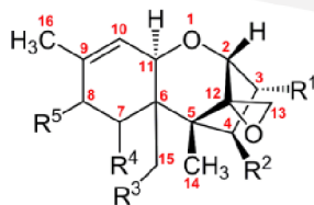
Trichotecen
