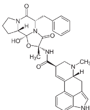
Obrázek 22: Ergotamin
