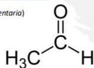
Acetaldehyd
