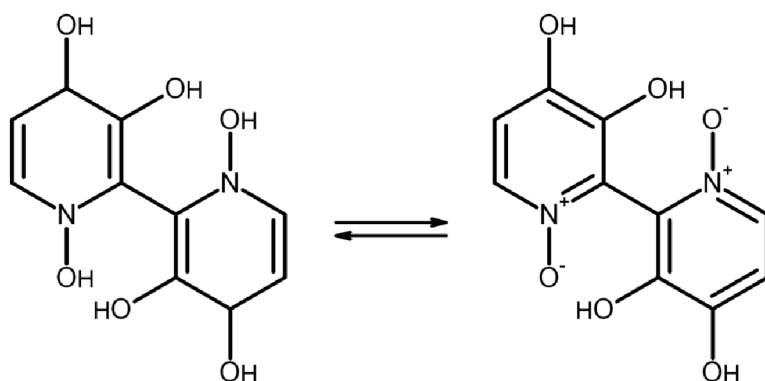
Obrázek 9: Orellanin
