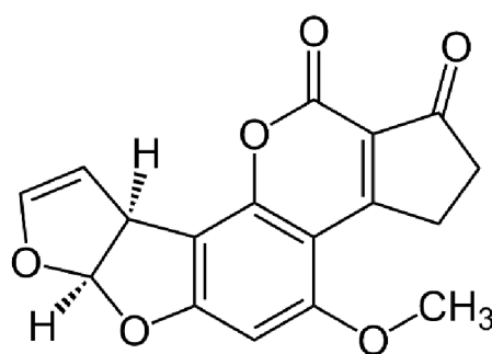
Obrázek 19: Aflatoxin B1
