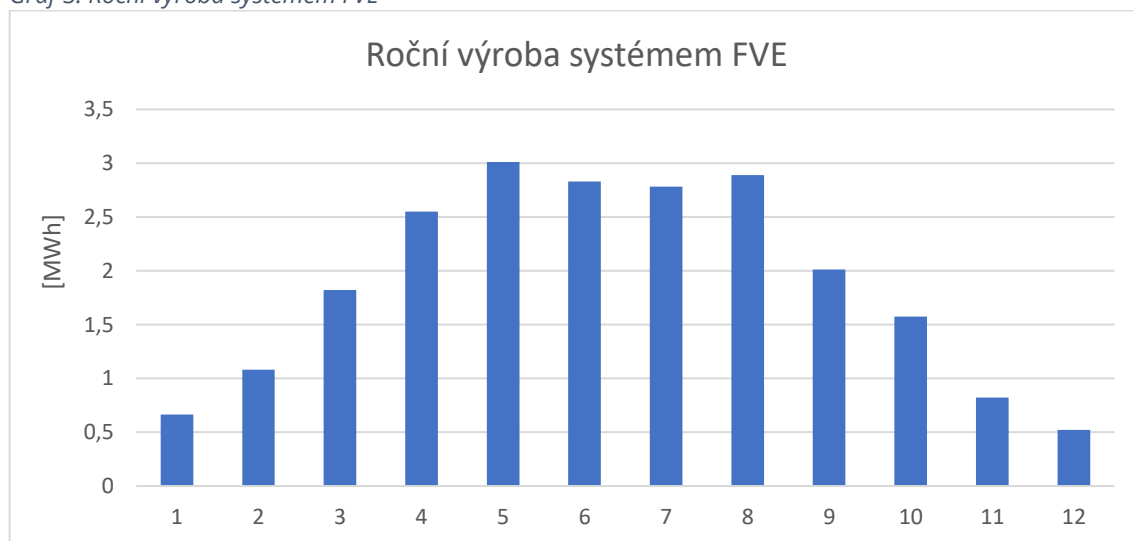
Graf 3: Roční výroba systémem FVE
