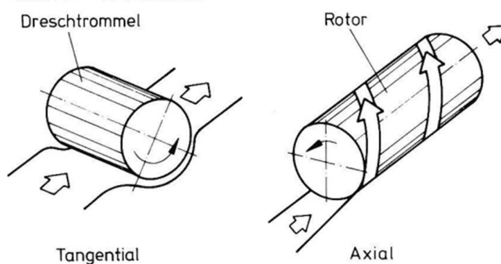
Obrázek 1.3: Tangenciální a axiální mlátící ústrojí (Michael Štelcl, 2014)
