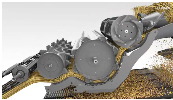
Obrázek 1.7: Dvoububnové mláticí ústrojí Claas APS (Claas.cz, 2024)
