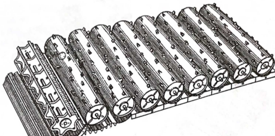
Obrázek 1.11: Rotační vytrásadlo (Kroupa, Hůla a Kovaříček, 2002)
