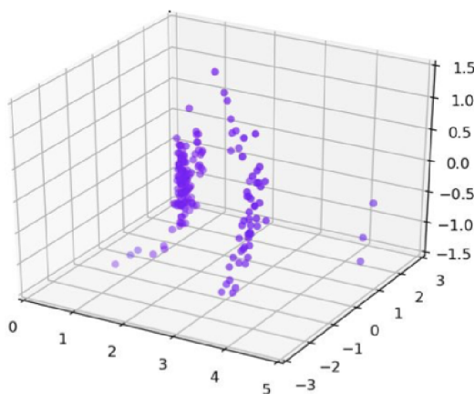
Obr. 3.8: Bodové mračno 2
