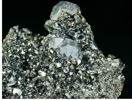
sfalerit[23]
