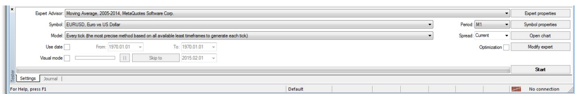
Obrázek 2.2: Tester strategií
