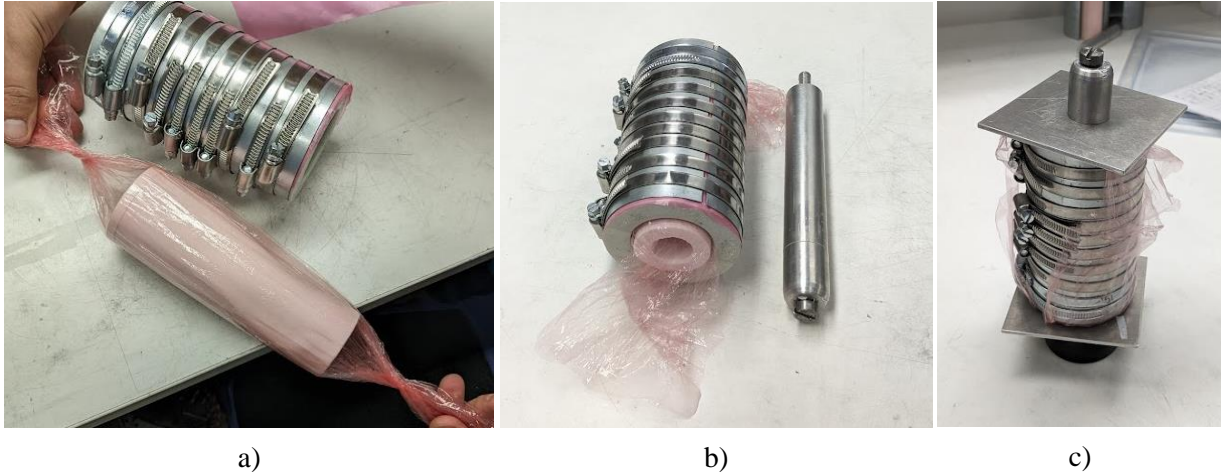
Obr. 14 Příprava formy pro lisování pomocí silikonového jádra.
