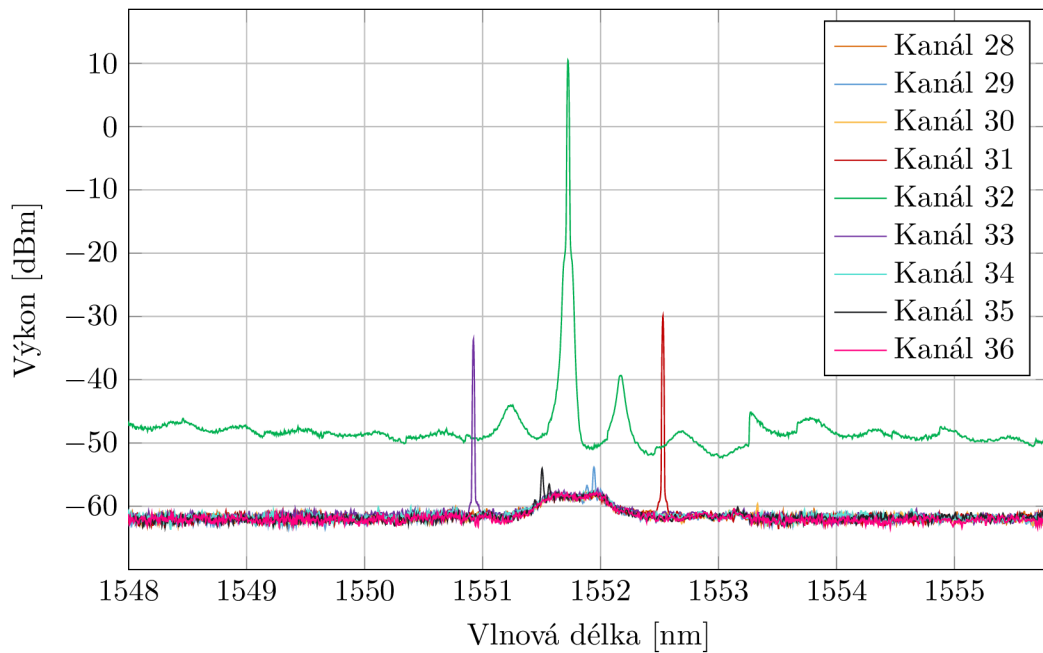
Spektrum pro zapojení: Filtr 1, PASS → COM
