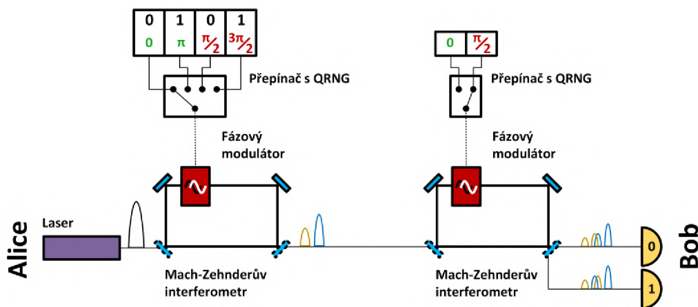
Obr. 2.4: Možná implementace protokolu BB84 s fázovým kódováním [27].
