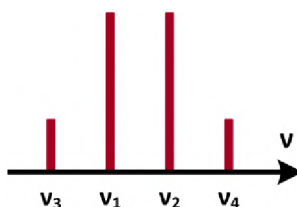
Obr. 7.9: Rozložení původních a nových frekvencí vzniklých důsledkem FWM [98].
