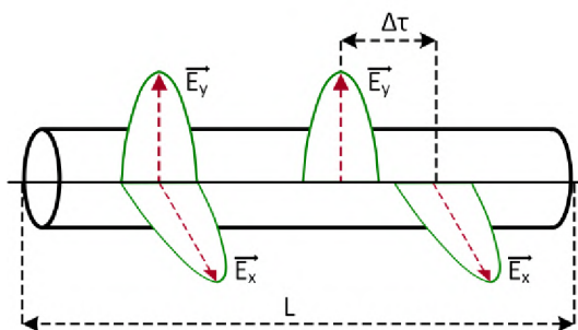
Obr. 7.6: Změna polarizace zapříčiněná PMD v optickém vlákně [67].
