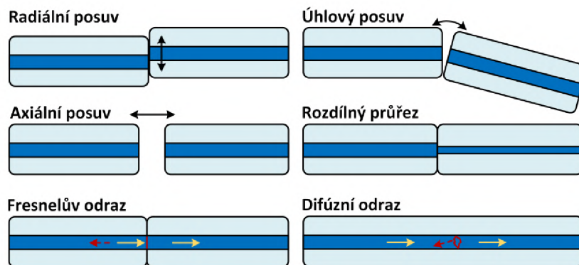
Obr. 7.2: Příčiny vzniku ztrát [67].
