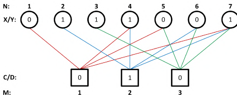
Obr. 3.1: Tannerův graf znázorňující výše uvedenou Gallagerovu matici.
