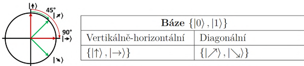
Obr. 2.1: Polarizační kódování.
