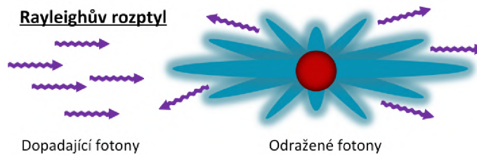
Obr. 7.10: Rayleighův rozptyl [106].
