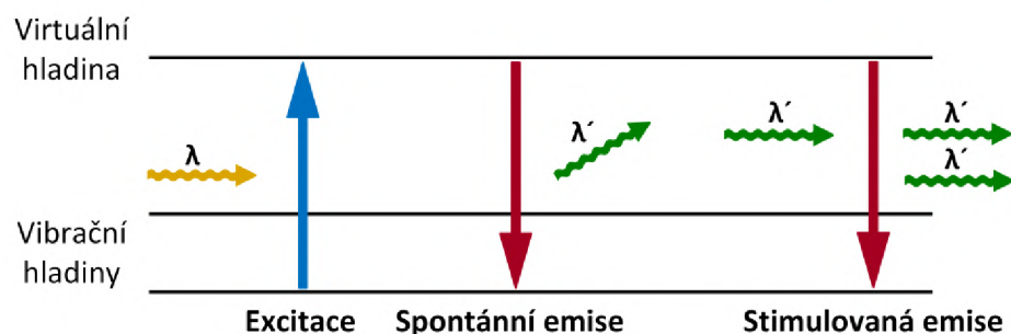
Obr. 7.7: Spontánní a stimulovaná emise [90].
