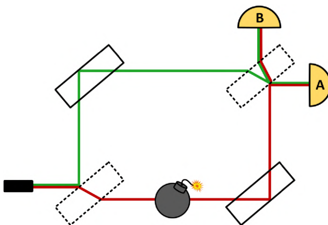
Obr. 5.1: Test funkčnosti bomby pomocí měření bez interakce.
