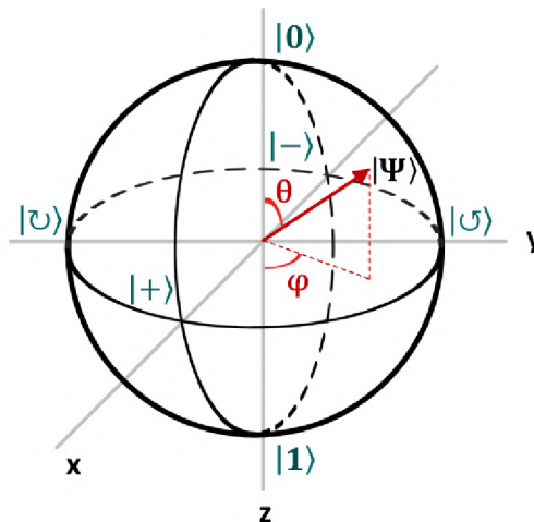
Obr. 1.7: Blochova koule [20].
