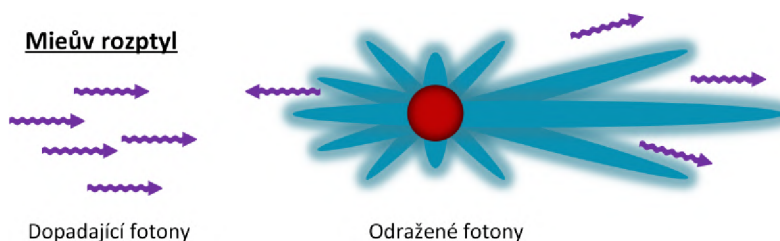
Obr. 7.11: Mieův rozptyl [106].
