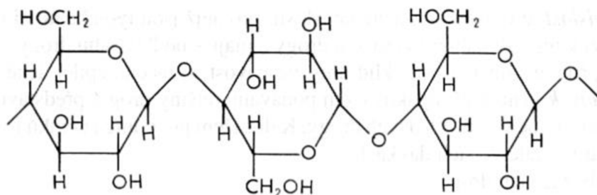
Celuloza (polysacharid)
