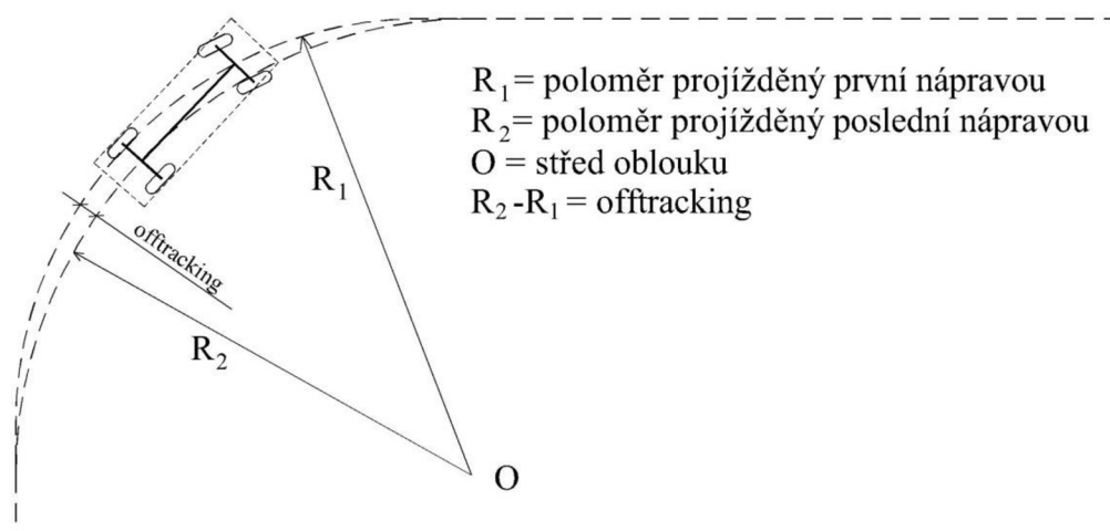
Obrázek 4 - Offtracking
