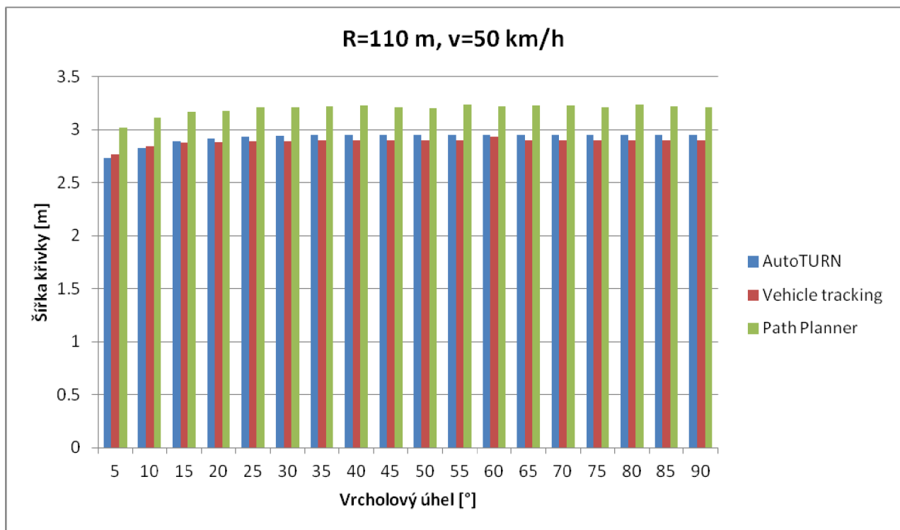
Graf 4 - Porovnání šířky vlečných křivek z různých programů (R=110 m, v=50 km/h)
