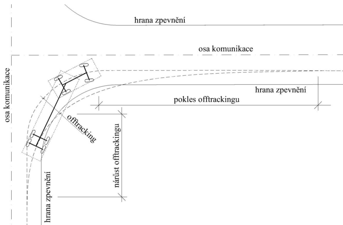
Obrázek 5 – Návěsová souprava při průjezdu směrovým obloukem malého poloměru
