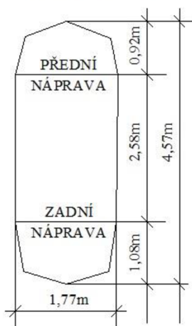
Obrázek 13 - Rozměry měřicího a simulovaného vozidla
