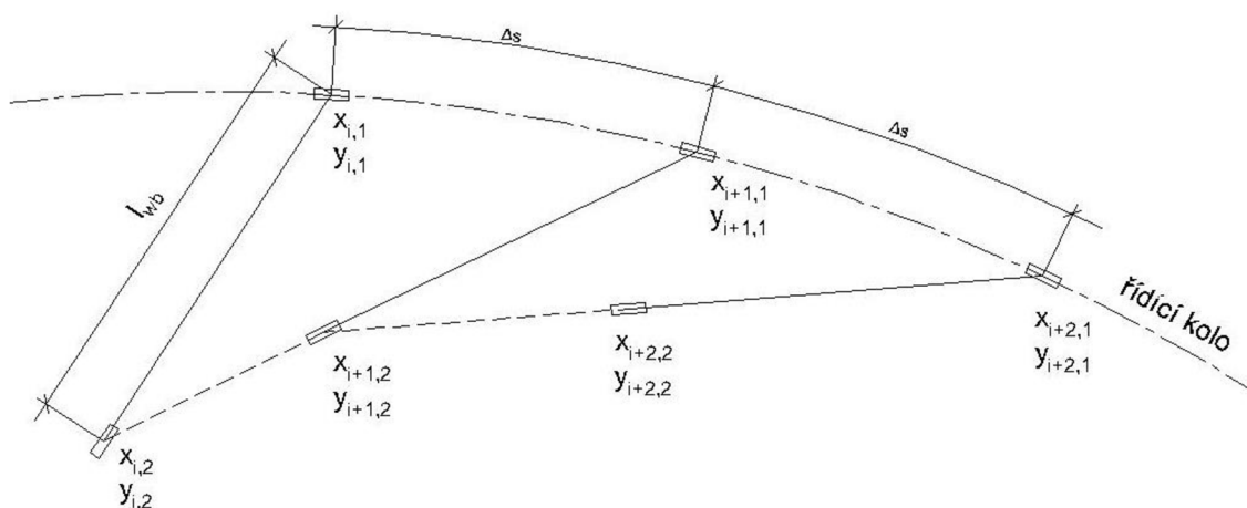
Obrázek 6 - Schéma výpočetního modelu jízdního kola
