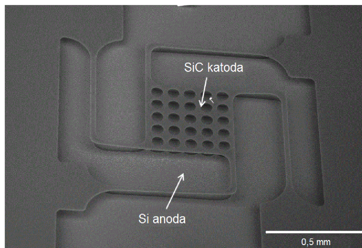
Obr. 29 Termoemisní generátor vyrobený technologií pro MEMS (upraveno z [45])
