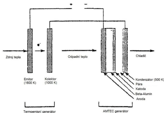
Obr. 19 Schéma kombinace termoemisního a AMTEC generátoru (upraveno z [33])
