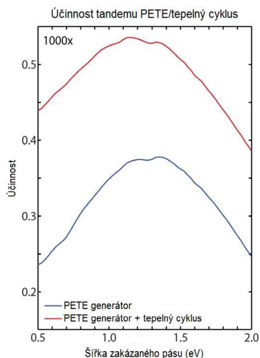
Obr. 28 Porovnání účinnosti PETE generátoru a tandemu PETE/tepelný cyklus (upraveno z [44])
