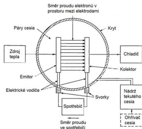
Obr. 9 Schéma cesiového termoemisního generátoru (upraveno z [1])
