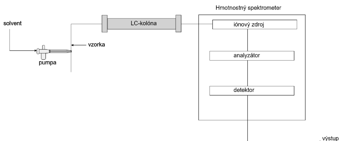
Obr. 5 Schéma LC-MS
