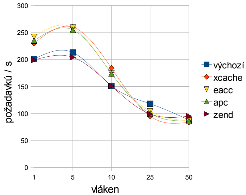
Graf 33: Výkon při použití PHP akceleratorů - 3
