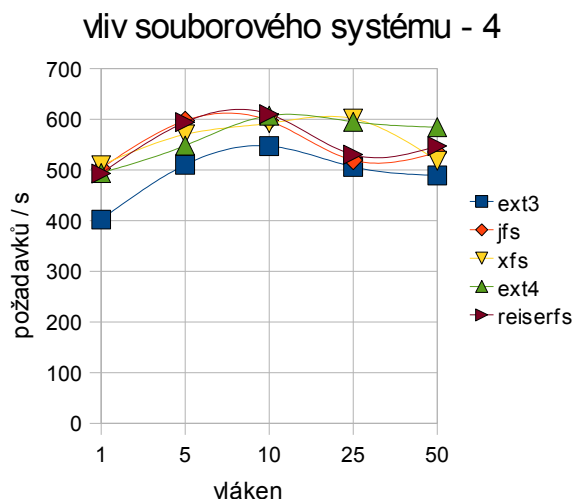
Graf 9: Vliv použitého filesystému
