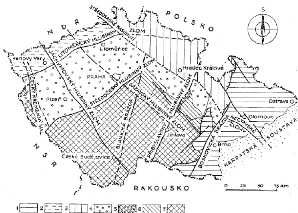
Obr. 1 Mapka předplatformních jednotek Českého masívu; 1 moravskoslezská oblast, 2 krušnohorská oblast, 3 lugická oblast, 4 středočeská oblast, 5 hlinská zóna středočeské oblasti, 6 kutnohorská-svratecká oblast, 7 moldanubická oblast (Mísař a kol. 1983).
