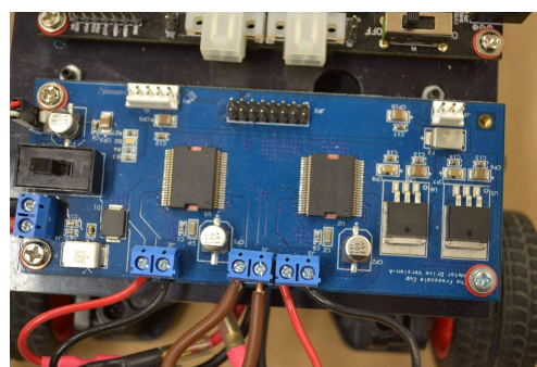
(b) Podpůrná (výkonová) deska plošných spojů
