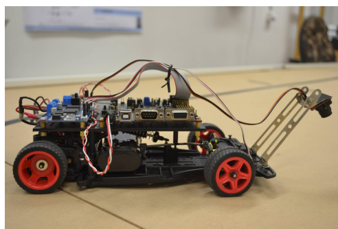
(b) Vozítko – pohled ze strany
