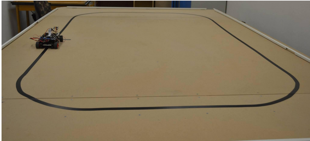
Obrázek 3.11: Testovací trať
