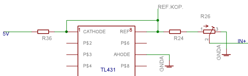
Obrázek 12 Zdroj referenčního napětí
