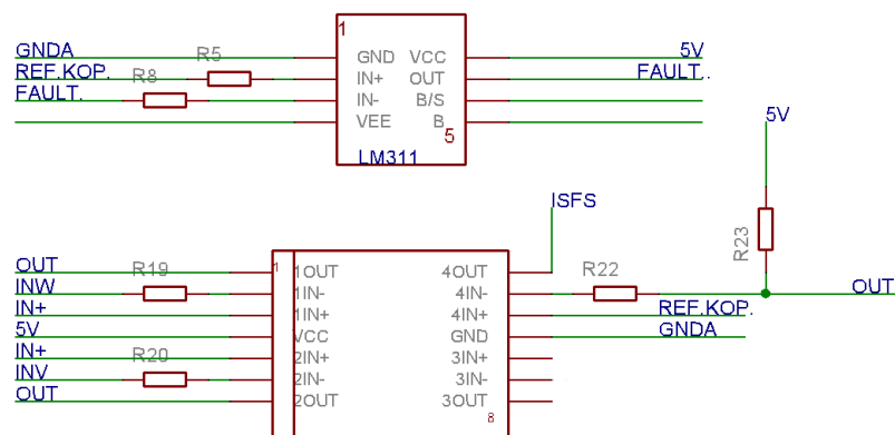
Obrázek 11 Pomocné obvody
