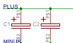
Obrázek 17 Stejnosměrný meziobvod
