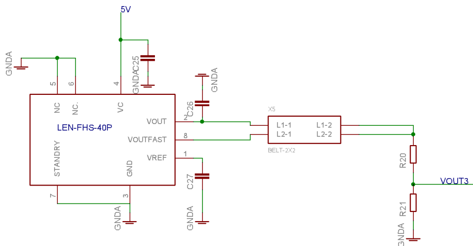
Obrázek 13 Obvod měření proudu
