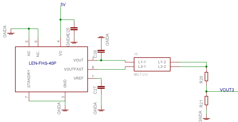
Obrázek 20 Měření proudu
