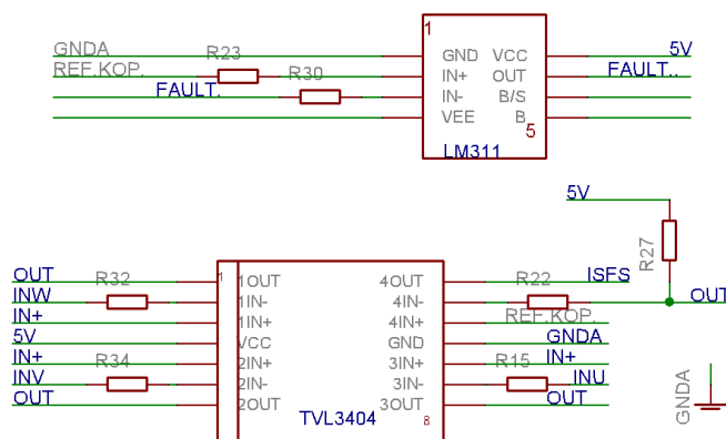
Obrázek 18 Pomocné obvody
