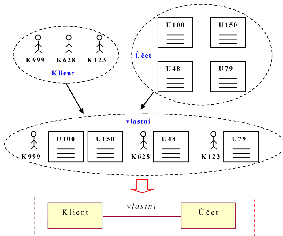
Obr. 2.3: Proces tvorby ER diagramu.
