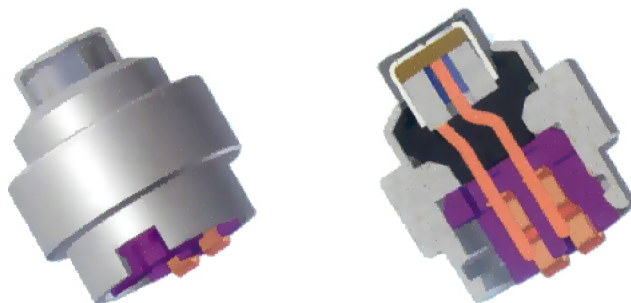
Obrázek 4.1: Load limiter
