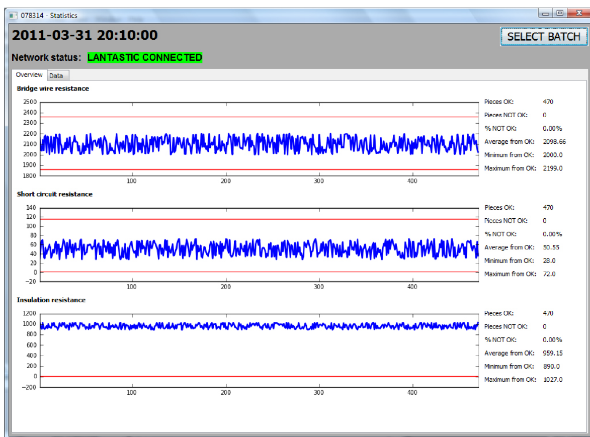
Obrázek 5.2: Hlavní obrazovka programu na vyhodnocování
