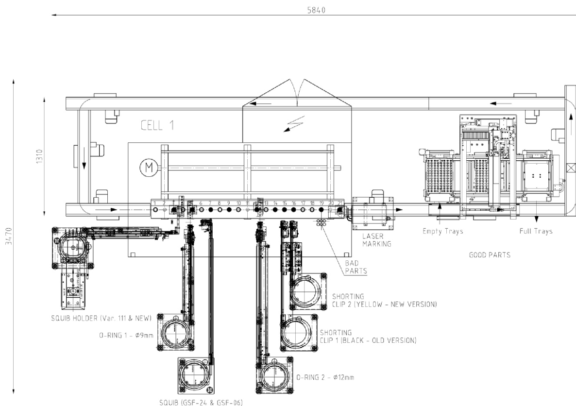
Obrázek 4.3: Linka Flexcell - pohled shora
