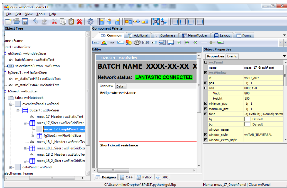
Obrázek 5.5: prostředí wxFormBuilderu
