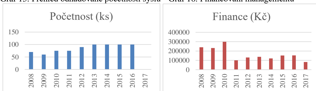
Graf 15: Přehled odhadované početnosti sysslů Graf 16: Financování managementu
