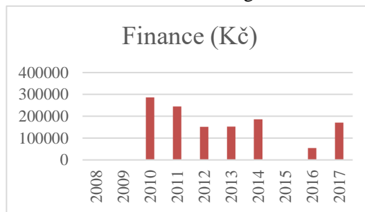
Graf 21: Přehled odhadované početnosti syslů Graf 22: Financování managementu
