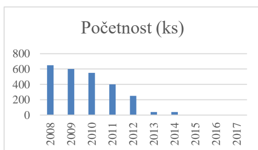
Graf 25: Přehled odhadované početnosti sýslů
