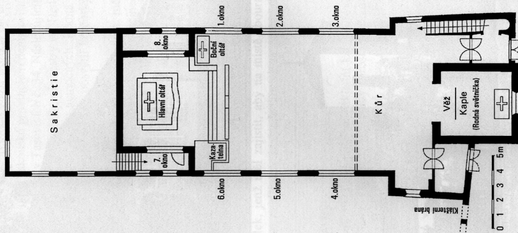
Půdorys kostela
