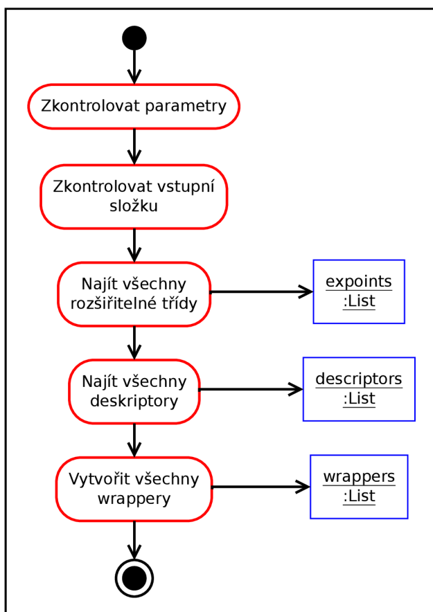
Obrázek 7.2: Diagram aktivit znázorňující běh programu PWM.
