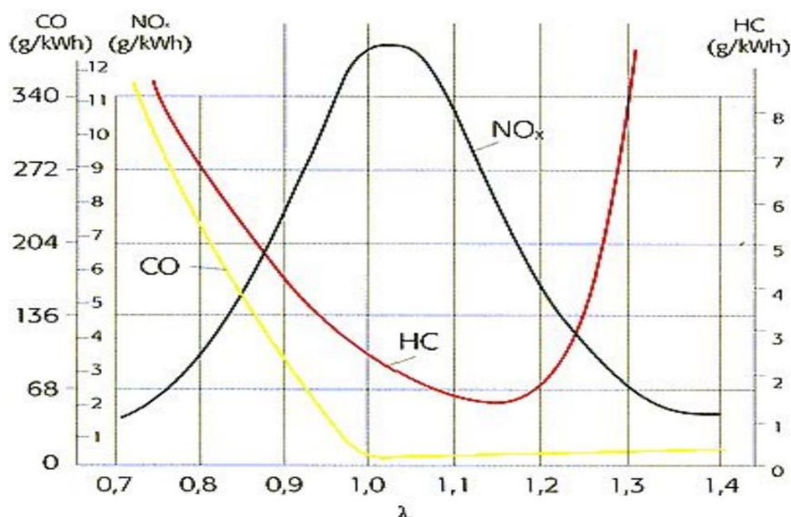
Obrázek 1 Vznik škodlivin v závislosti na přebytku vzduchu pro zážehový motor [5]
