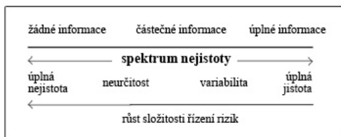
Obrázek 1 Spektrum nejistoty
