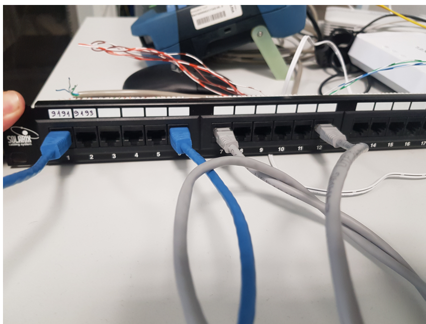
Obr. A.1: Zapojení patch panelu pro simulaci vzdálenosti 100 metrů
