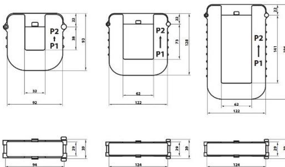
Obrázek 9.: Rozměry pevného dělitelného transformátoru na pásoviny [12]
