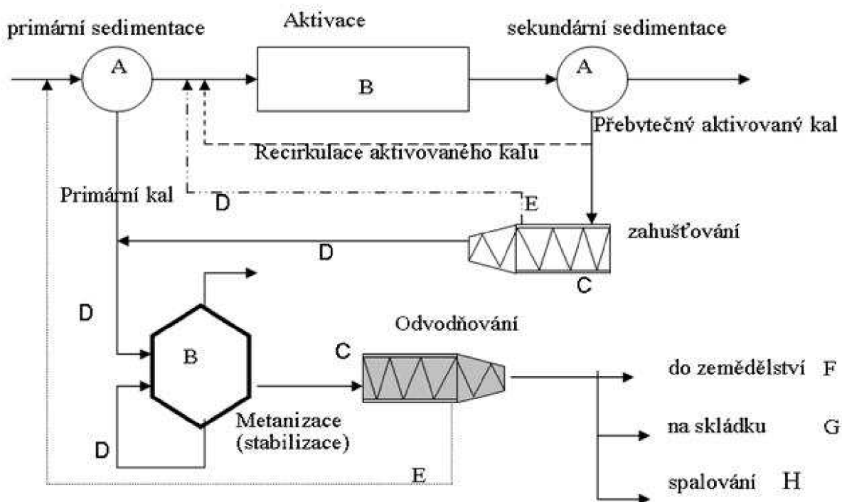
Obrázek 2-2 Základní schéma kalového hospodářství na ČOV [3]
