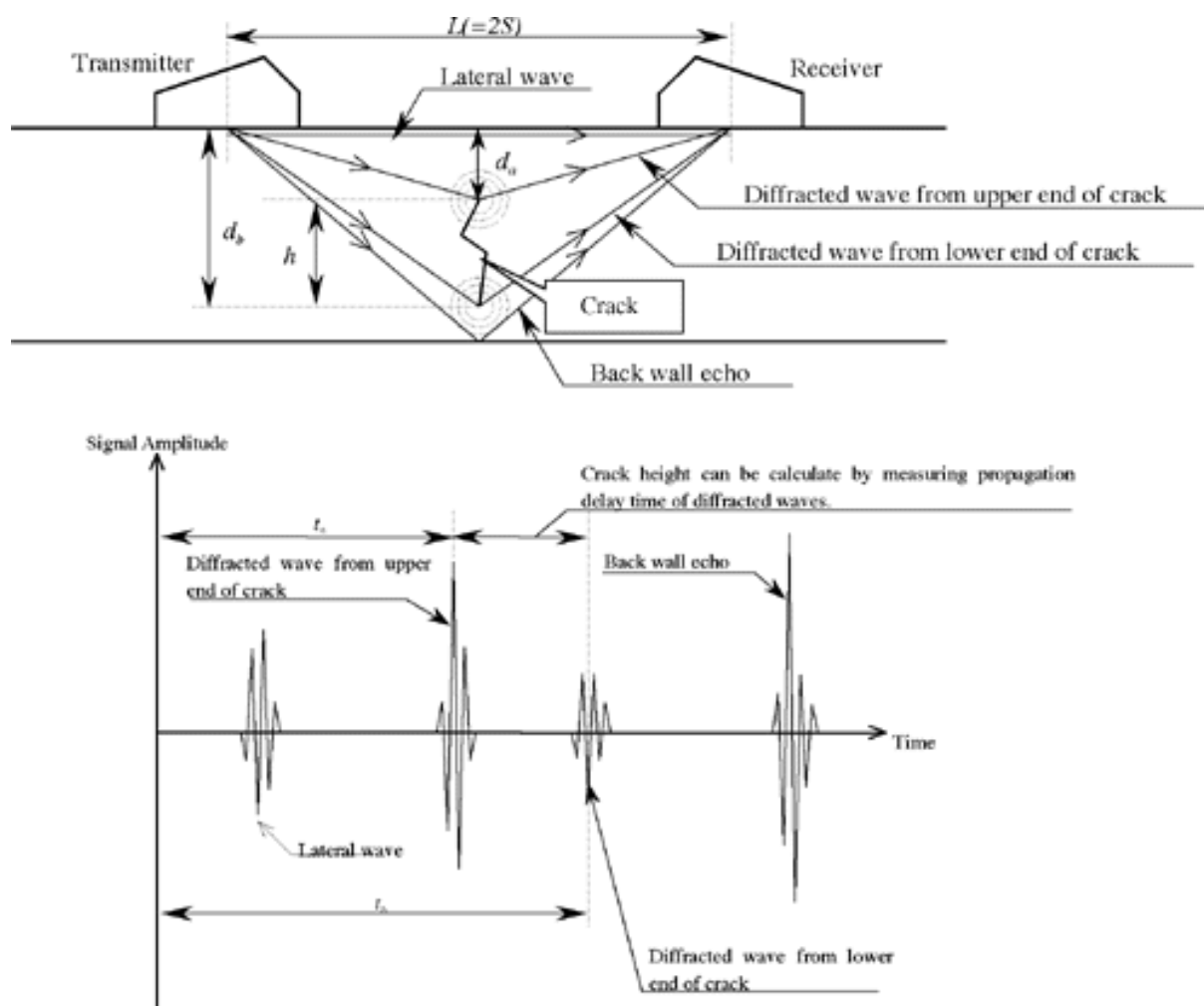
Obr. 10 Metoda zobrazení TOFD[15]
