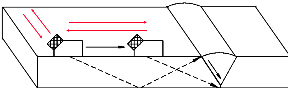
Obr. 8 Metody zkoušení – přímé a podélné [13]
