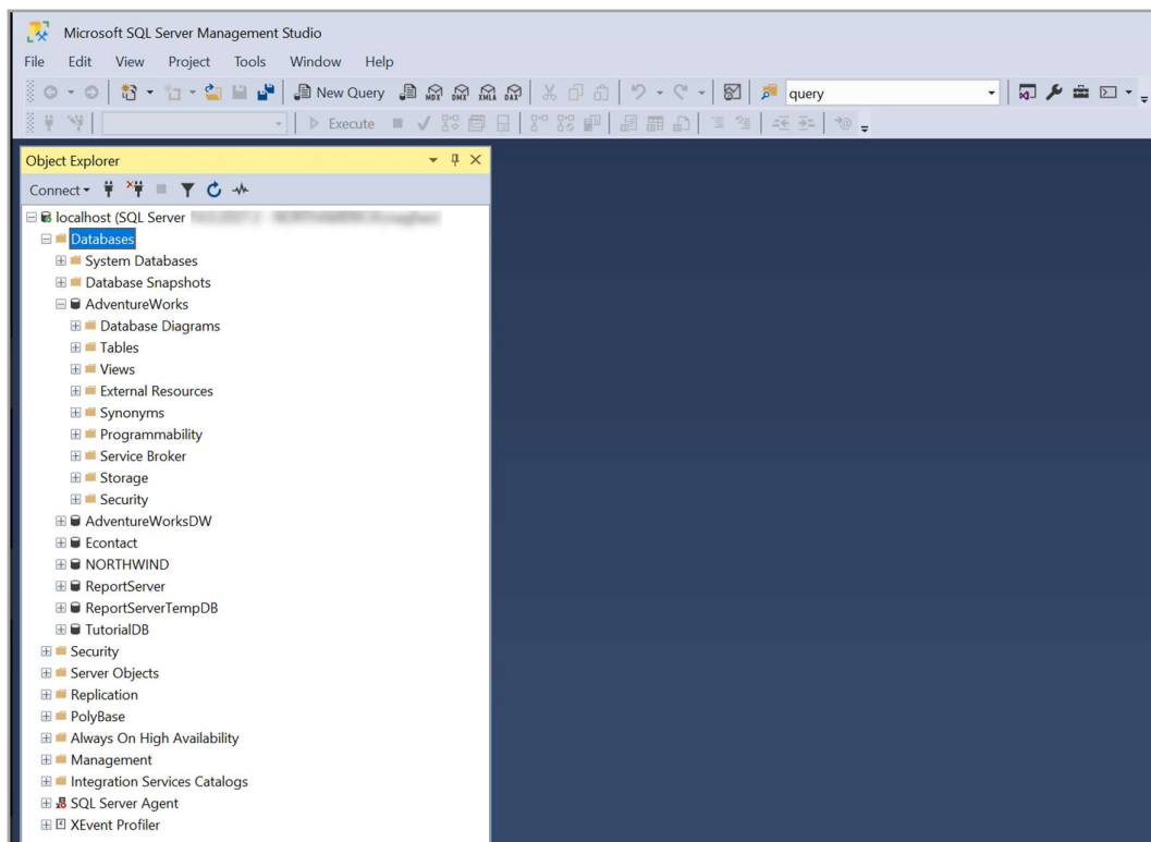
Obrázek 19: Ukázka SSMS [29]
