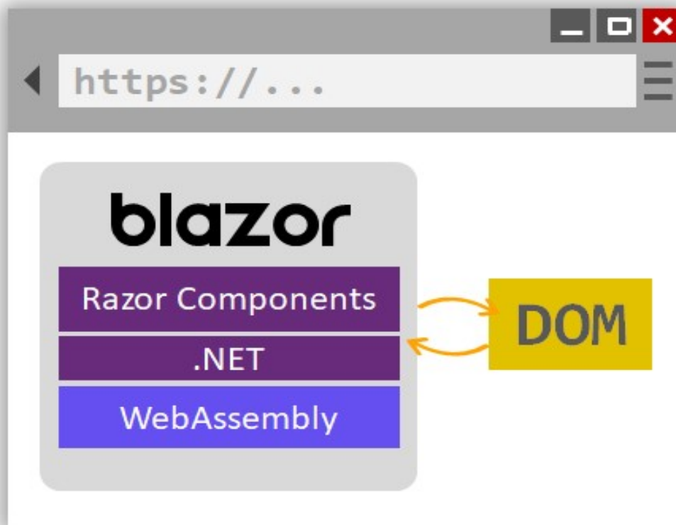
Obrázek 28: Struktura WebAssembly [50]
