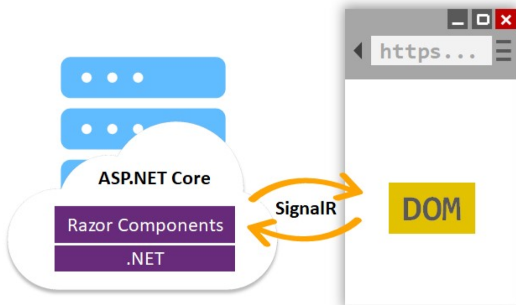
Obrázek 29: Struktura Blazor Server [50]
