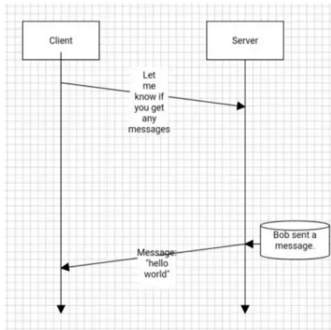
Obrázek 11: Znárodnění komunikace mezi klientem a serverem u WebSocketu. Zdroj: [33]
