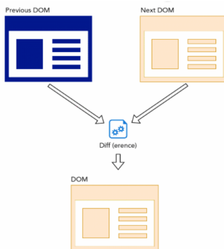
Obrázek 6: Princip fungování virtuálního objektového modelu dokumentu. Zdroj: [18]
