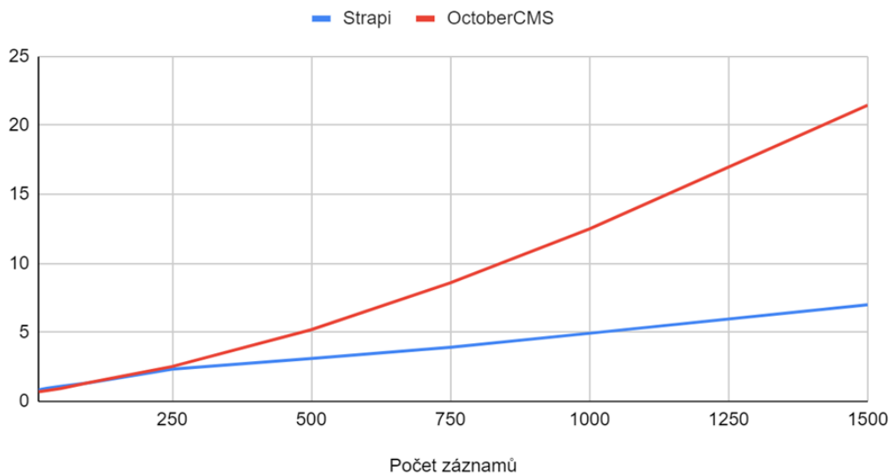
Obrázek 6 - Graf Strapi vs October CMS
