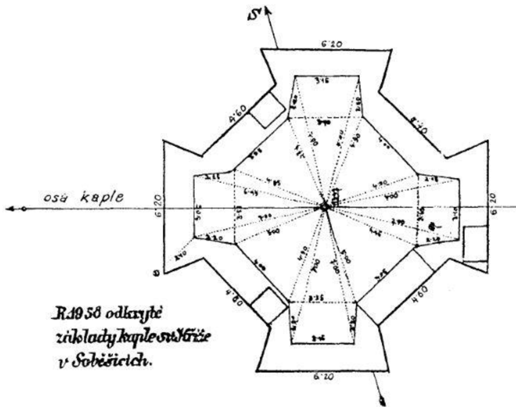
Obr. 17: Půdorys kaple
