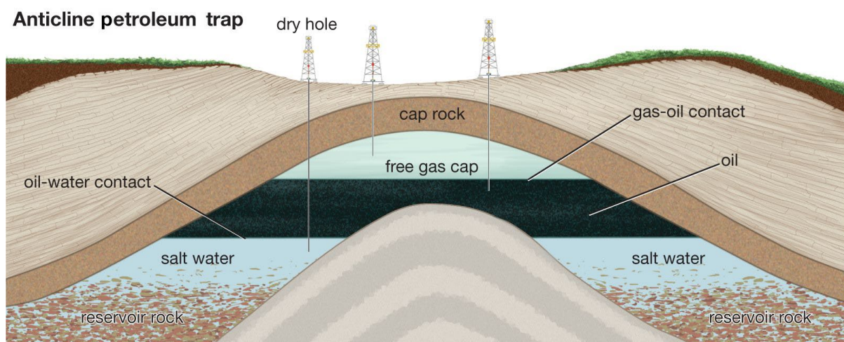
Obrázek 2: Antiklinární strukturní past
