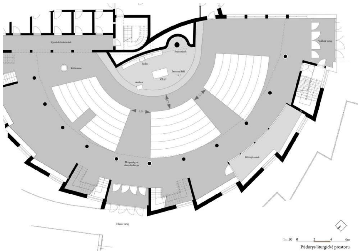
7. Jiří Štásta, půdorys presbytáře. Soukromý archiv, Jiří Štásta.
