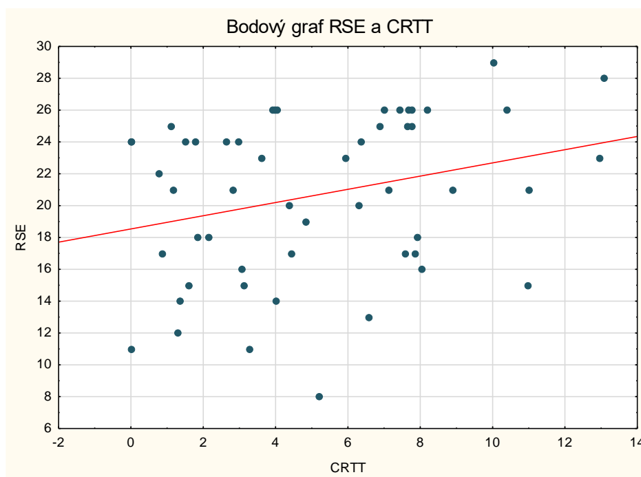
Obrázek 9. Bodový graf RSE a CRTT
