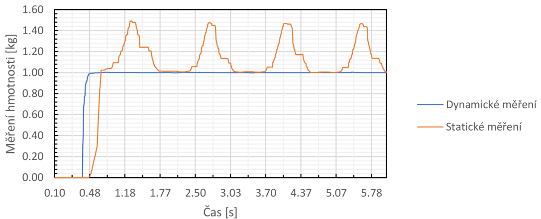
Obrázek 4.5: Porovnání způsobů měření hmotnosti závaží
