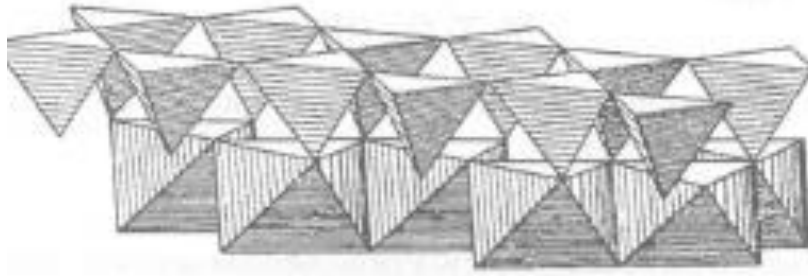
Obr. 7: Grafické znázornění vrstvy typu 1:1. [5]
