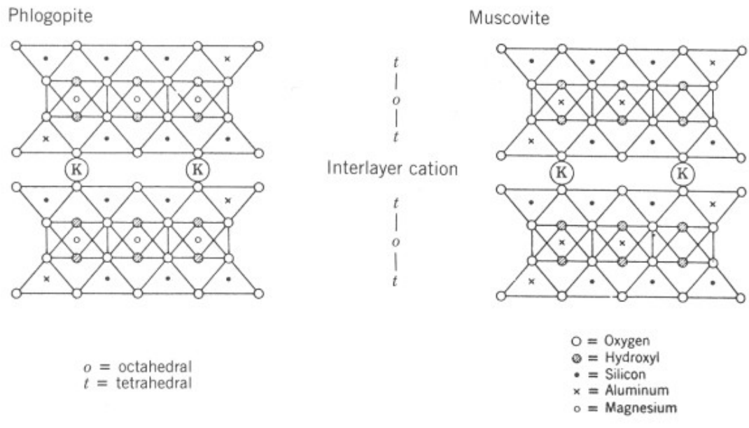
Obr. 12: Znárodnění kationtů v mezivrstvě minerálů skupiny slíd. [5]
