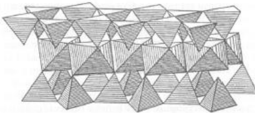
Obr. 8: Grafické znázornění vrstvy typu 2:1. [5]
