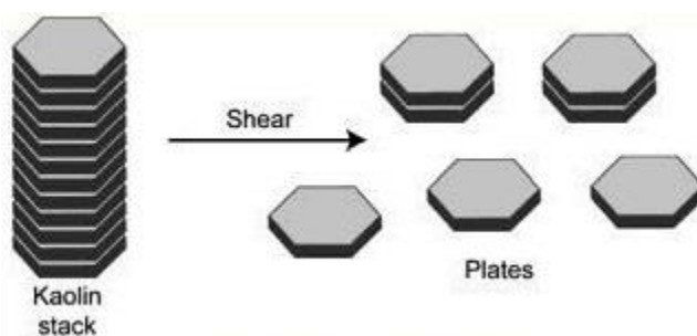
Obr. 40: Delaminace kaolinitu.[27]
