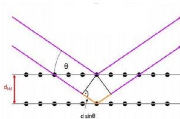
Obr. 32: Grafické znázornění Braggovy rovnice.[50]
