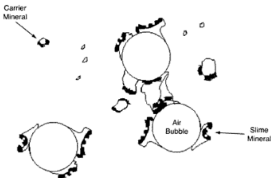
Obr. 20: Schéma plavení s nosnými částicemi. [29]
