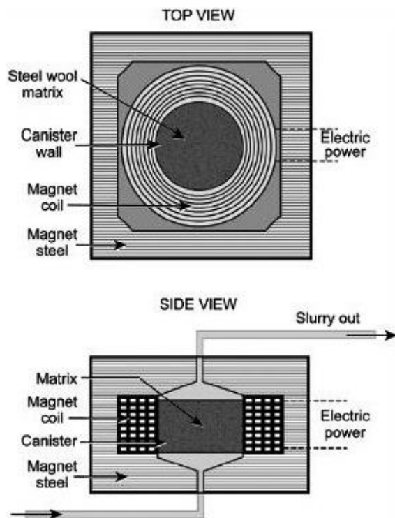
Obr. 22: Schéma magnetického separátoru s magnetem o intenzitě 2 T. [27]
