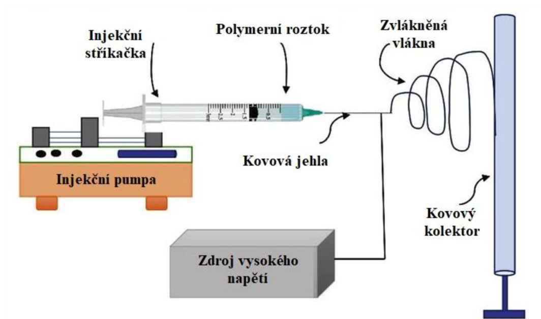
Obrázek 9: Schéma elektrostatického zvlákňování z jehly, převzato a přeloženo z (26)
