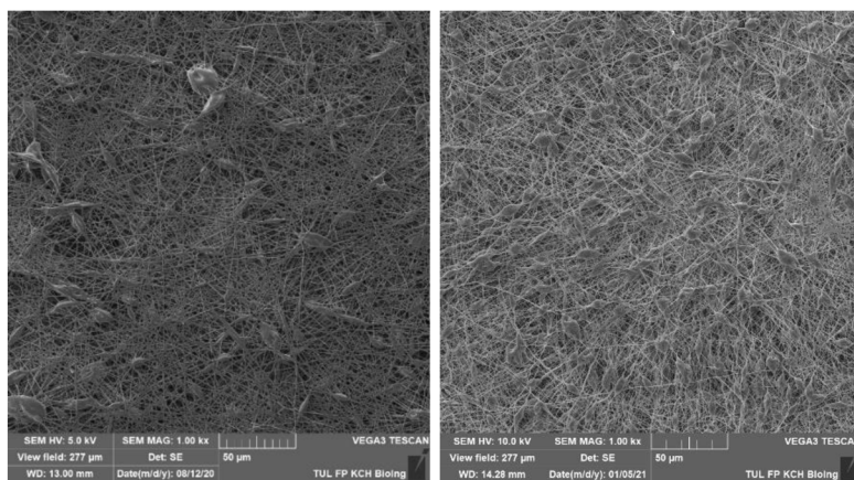
Obrázek 17: Vybrané SEM snímky zvlákněné struktury vzorku č. 5, 1. den vlevo a 2. měsíc vpravo, měřítko je 50 mikrometrů
