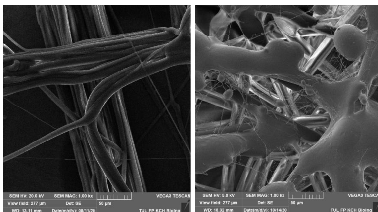
Obrázek 14: Vybrané sem snímky zvlákněné struktury vzorku č. 2, 0. den vlevo a 7. den vpravo, měřítko je 50 mikrometrů
