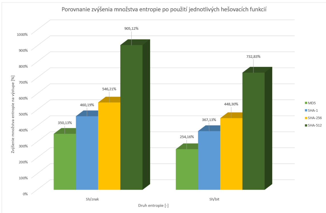
Obr. 4.3: Porovnanie zvýšenia množstva entropie po použití jednotlivých hešovacích funkcií.
