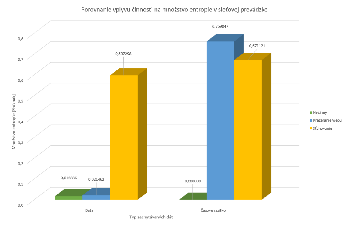
Obr. 4.2: Porovnanie vplyvu činnosti na množstvo entropie v sieťovej prevádzke.
