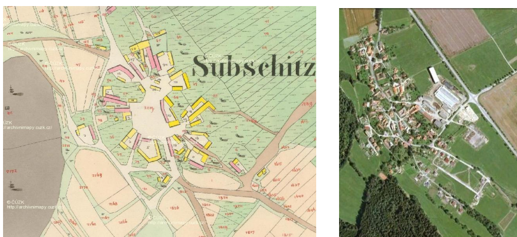
Mapa 1. Vývoj rozlohy sídla Zubčice v letech 1827 a 2009
