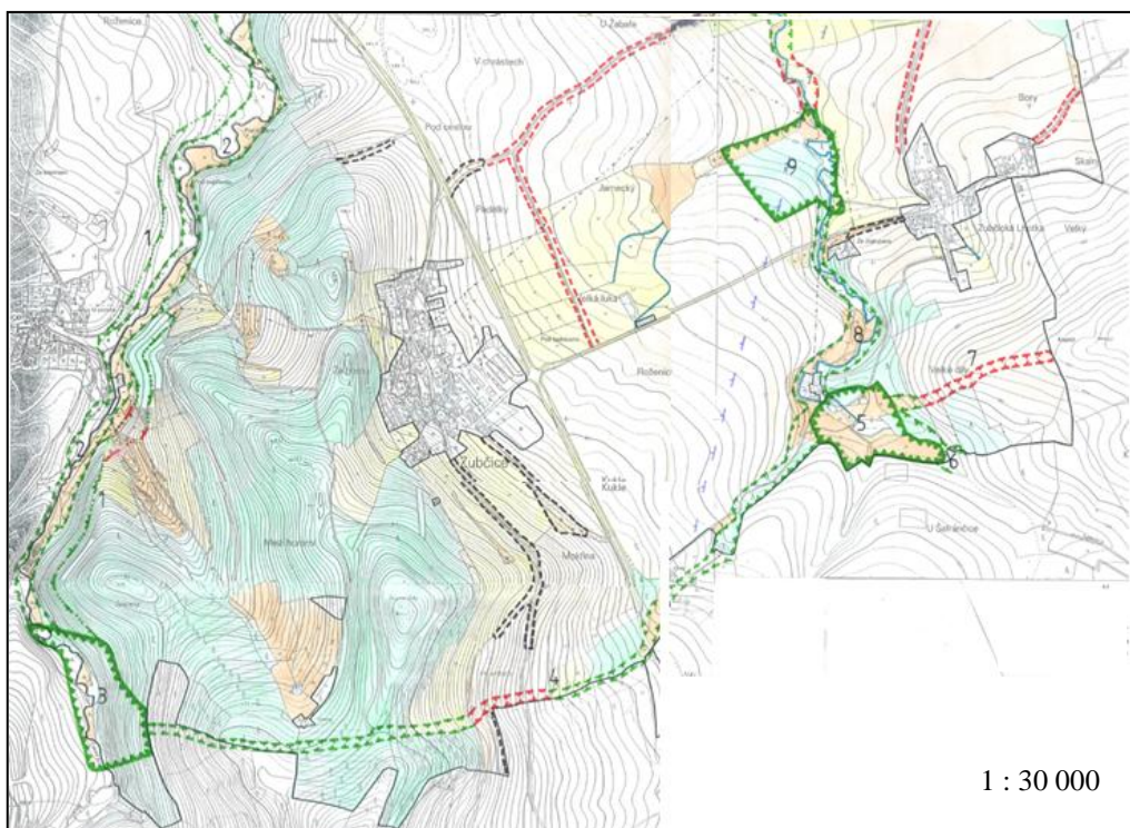
Obr. 3. Plán místního ÚSES pro Zubčice, Markvartice a Zubčickou Lhotku (okolí sídel Zubčice a Zubčická Lhotka)
