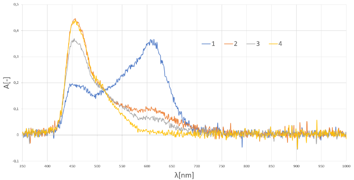
Obr. 6.28: Graf závislosti absorpce na vlnové délce u měření tvrdosti vody (spektrofotometr)
