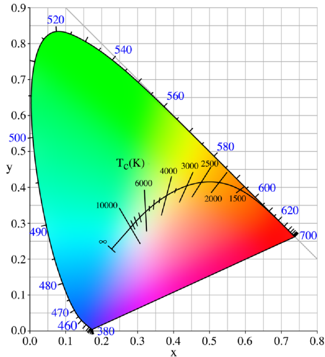
Obr. 2.4: Kolorimetrický trojúhelník [5]
