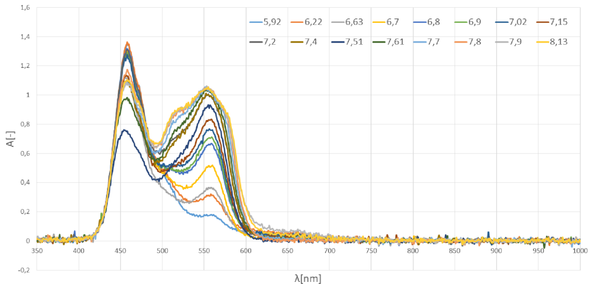
Obr. 6.5: Graf závislosti absorpance na vlnové délce u fenolové červeně (spektrofotometr)
