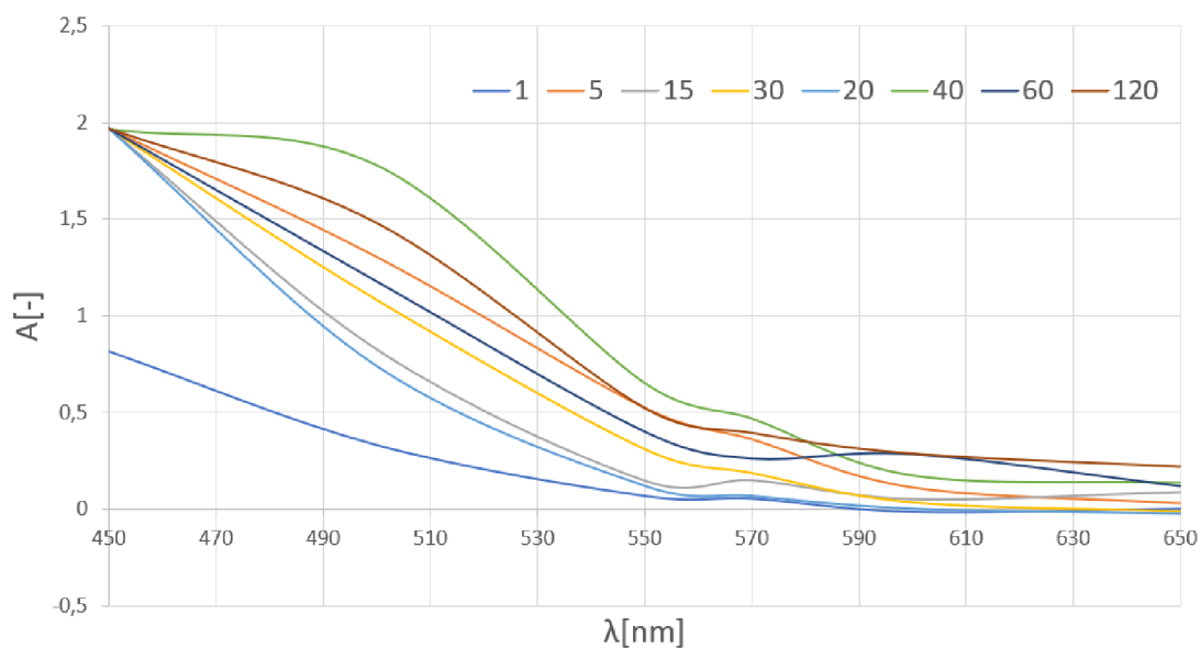
Obr. 6.23: Graf závislosti intenzity světla na vlnové délce u koncentrace dusičnanů (senzor)
