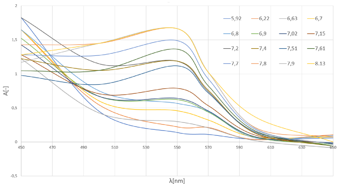
Obr. 6.7: Graf závislosti absorbance na vlnové délce u fenolové červeně (senzor)
