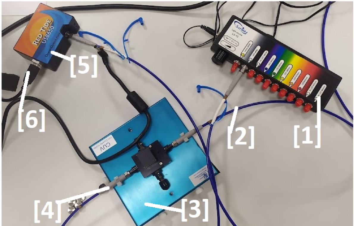
Obr. 4.9: Realizace měřicí sestavy se spektrofotometrem
