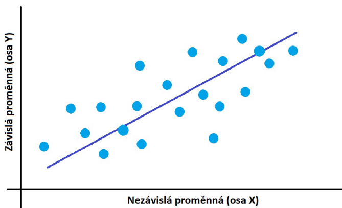
Obr. 3.1: Model jednoduché lineární regrese
