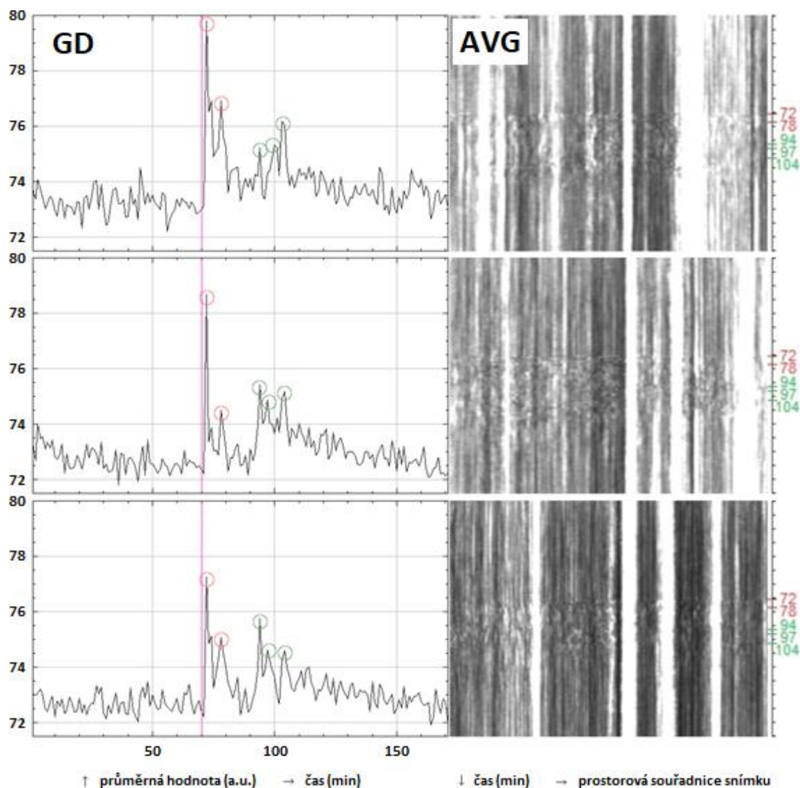
Obr. 18 Analýzy změn struktury koherenční zmitosti po lokálním vysokoteplotním stresu vzorku provedené s využitím obrazových metod GD ( levý sloupec ) a AVG ( pravý sloupec ). Horní panel obrázku odpovídá oblasti zájmu nejbližší místu popálení, prostřední panel obrázku odpovídá střední oblasti zájmu a dolní panel obrázku odpovídá oblasti zájmu nejdále od místa popálení (viz obr. 11 a obr. 12). Analýzy vzorku s využitím metody GD jsou prezentovány ve formě grafů závislosti hodnot PZSKZ příslušných dané oblasti zájmu (vertikální osy) na čase pořizování jednotlivých sérií snímků struktur KZ (horizontální osa). Růžové čáry vyznačují okamžik popálení vzorku topným tělesem. Analýzy vzorku s využitím metody AVG (pravý sloupec) jsou prezentovány ve formě map THSP, kde vertikální rozměr představuje čas pořizení příslušné série snímků struktur KZ a horizontální rozměr představuje prostorovou souřadnici vypočtených výsledných snímků v oblasti zájmu (viz obr. 12). Červeně jsou ve schématu vyznačeny iniciální skokové změny struktur vzorků v reakci na tepelný stres, zeleně jsou vyznačeny sekundární skokové změny struktur vzorků detekované s časovou prodlevou po iniciálních změnách. Skokové změny struktur vzorků se v analýze metodou GD projevují jako vrcholy, v analýze metodou AVG jako změna zmitosti v mapách THSP. Měření 1/7.
