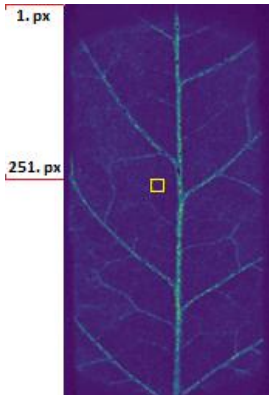
Obr. 10 Oblast zájmu (viz žlutý čtverec ) zvolená ve snímcích struktury koherenční zrnitosti ( 584 \times 568 px) pro účel analýzy souvislostí změn ve struktuře koherenční zrnitosti s pohybem chloroplastů. První (horní) řádek oblasti zájmu (žlutý čtverec) byl pro všechna měření umístěn 251 px od horního okraje snímků struktur koherenční zrnitosti. Horizontální umístění oblasti zájmu bylo voleno pro každý list jinak, vždy s ohledem na rozmístění žilnatiny v pletivu konkrétního listu, s účelem zaměření opticky homogenní části pletiva k následné analýze.
