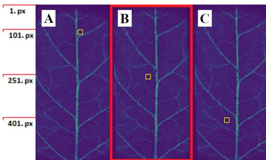
Obr. 25 Oblasti zájmu zvolené ve snímcích struktury KZ (viz žluté čtverce, A, B, C ) pro účel analýzy trendů PSKZ ve druhém ostrém experimentu. Detailní popis viz obr. 11. Oblast zájmu označená červeným rámečkem je totožná s oblastí zájmu použitou pro první ostrý experiment, a byly na ní porovnávány změny PSKZ ve zvolených intervalech z obou experimentů.
