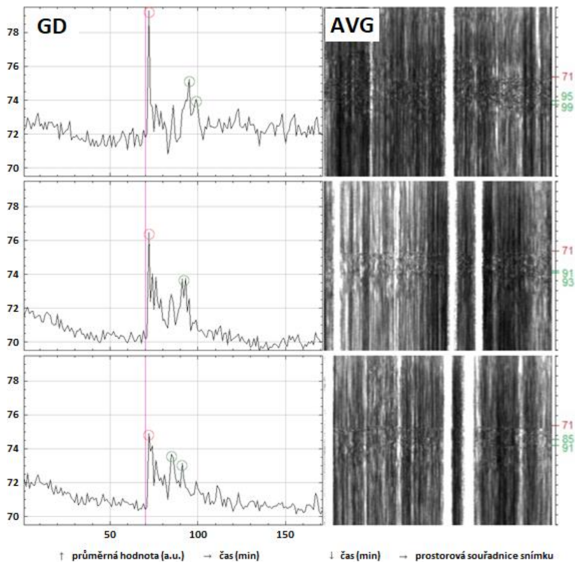
Obr. 23 Analýzy změn struktury koherenční zrnitosti po lokálním vysokoteplotním stresu vzorku provedené s využitím obrazových metod GD (levý sloupec) a AVG (pravý sloupec). Detailní popis viz legenda obr. 18. Měření 6/7.
