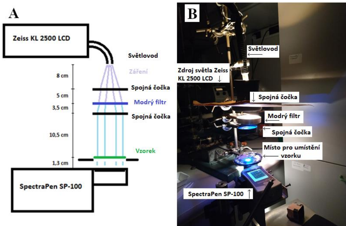
Obr. 9 Schéma měřicí aparatury pro pilotní experiment (A), fotografie měřicí aparatury pro pilotní experiment (B). A: Osa udává vzdálenosti mezi jednotlivými prvky aparatury. B: Záření ze zdroje (Zeiss KL 2500 LCD) je vyvedeno světlovodem nad vzorek. Paprsky záření dále prochází soustavou dvou kolimačních čoček a skrze modrý filtr až na vzorek. Rovnoběžně se vzorkem (listem) je do aparatury umístěn detektor (SpectraPen SP-100), jehož detekční plocha snímá vzorkem propuštěné paprsky záření v kolimovaném směru. Pilotní experiment byl realizován na pracovišti Katedry biofyziky UP.
