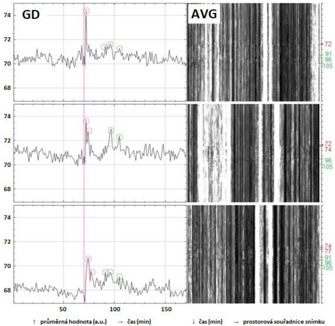
Obr. 22 Analýzy změn struktury koherenční zmitosti po lokálním vysokoteplotním stresu vzorku provedené s využitím obrazových metod GD (levý sloupec) a AVG (pravý sloupec). Detailní popis viz legenda obr. 18. Měření 5/7.
