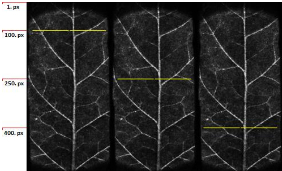
Obr. 12 Snímky struktur koherenční zrnitosti se zvolenými oblastmi zájmu (viz žluté úsečky ) použitých k analýze změn struktury koherenční zrnitosti po lokálním vysokoteplotním stresu metodou AVG. Všechny oblasti zájmu mají rozměry 230 \times 1 px. V levé části obrázku je oblast zájmu volená 100 px od horních okrajů snímků struktur KZ, v prostřední části obrázku je oblast zájmu volená 250 px od horních okrajů snímků skstruktur KZ, v pravé části obrázku je oblast zájmu volená 400 px od horních okrajů snímků skstruktur KZ. Horizontální umístění oblastí zájmu bylo pro každé měření voleno stejně.
