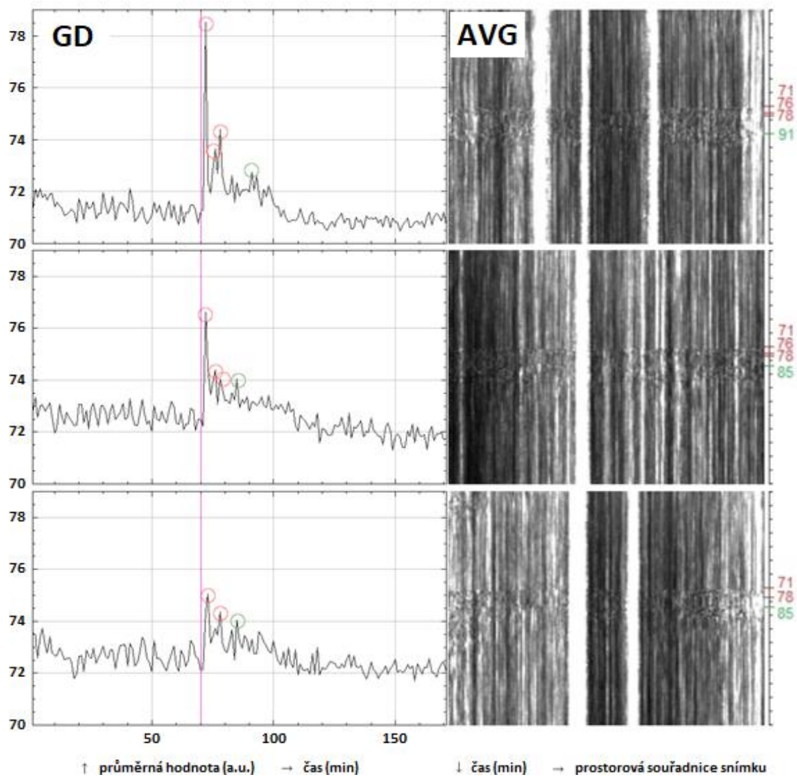
Obr. 21 Analýzy změn struktury koherenční zrnitosti po lokálním vysokoteplotním stresu vzorku provedené s využitím obrazových metod GD (levý sloupec) a AVG (pravý sloupec). Detailní popis viz legenda obr. 18. Měření 4/7.
