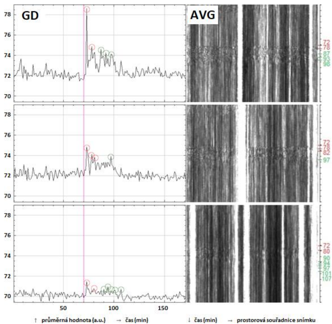
Obr. 20 Analýzy změn struktury koherenční zrnitosti po lokálním vysokoteplotním stresu vzorku provedené s využitím obrazových metod GD (levý sloupec) a AVG (pravý sloupec). Detailní popis viz legenda obr. 18. Měření 3/7.
