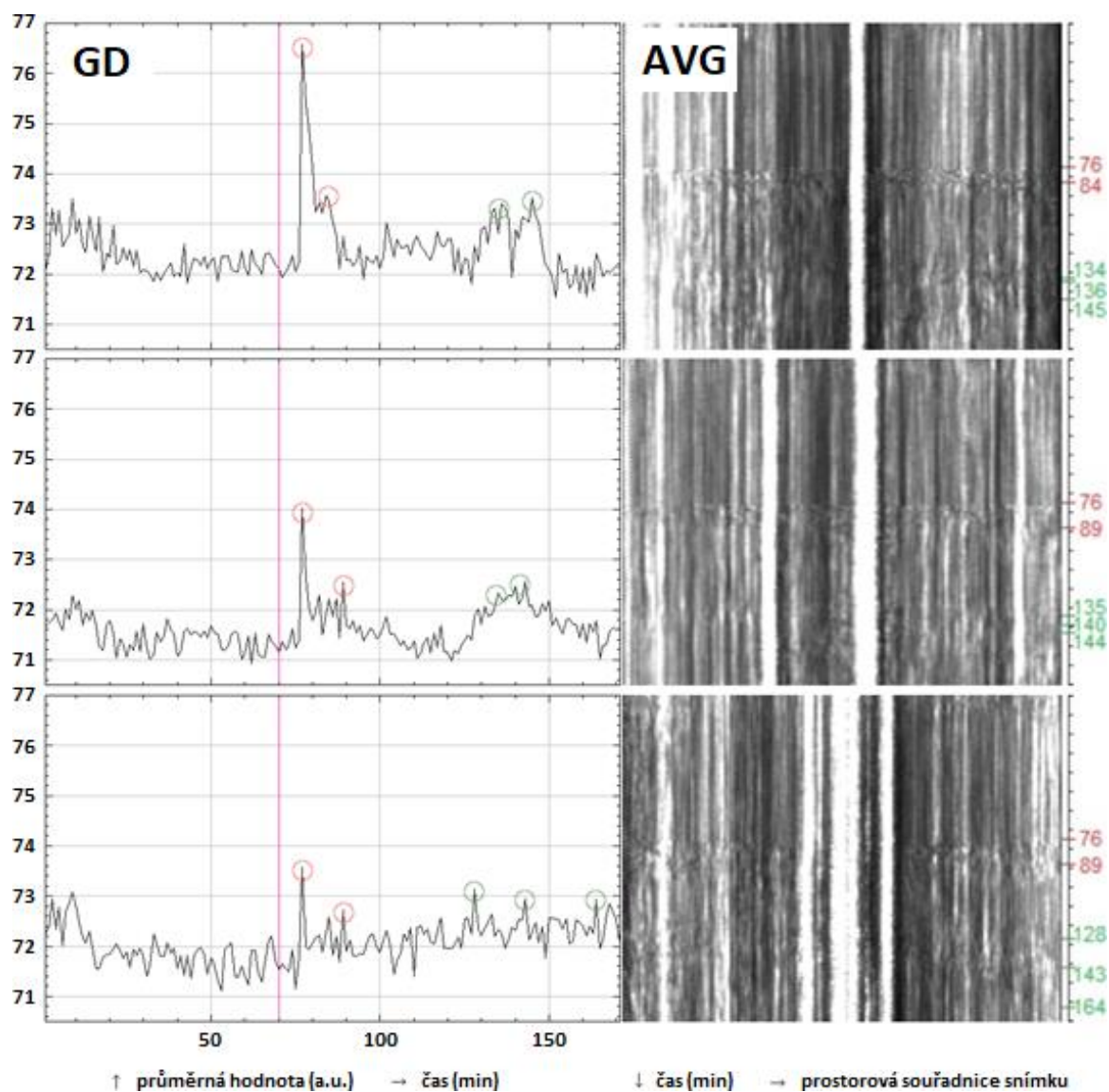
Obr. 19 Analýzy změn struktury koherenční zrnitosti po lokálním vysokoteplotním stresu vzorku provedené s využitím obrazových metod GD (levý sloupec) a AVG (pravý sloupec). Detailní popis viz legenda obr. 18. Měření 2/7.
