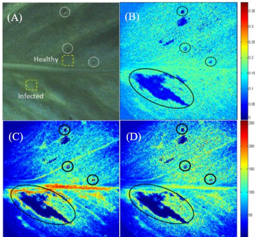
Obr. 2 Mapy struktury KZ v listu Epipremnum aureum : (A) fotografie listu s vyznačením zdravých a infikovaných (kolonizovaných) ploch, (B) obrazová analýza LASCA, (C) obrazová analýza Fujii, (D) obrazová analýza GD. Barevná stupnice odráží hodnoty BA. Modrá barva odráží nízkou úroveň pohybu v pletivu, červená barva představuje vysokou úroveň pohybu v pletivu (modifikováno z Ansari a kol. 2018).
