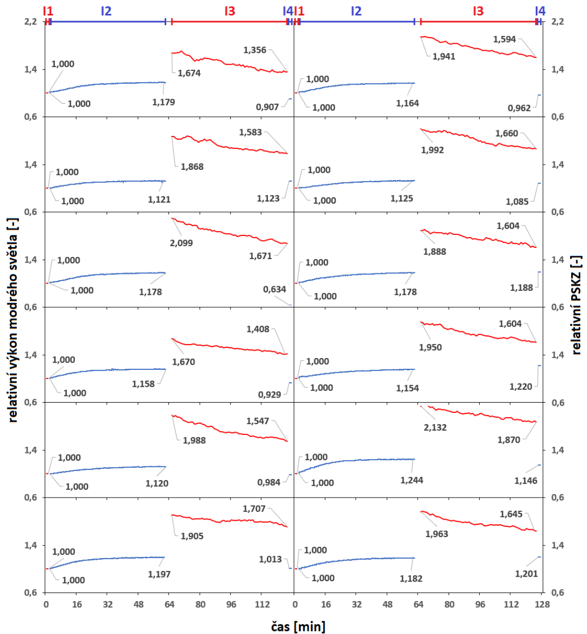
Obr. 16 Souvislosti změn ve struktuře koherenční zrnitosti s pohybem chloroplastů. Levá vertikální osa udává relativní výkon prošlého modrého světla vzorkem. Pravá vertikální osa udává relativní hodnoty PSKZ. Data označená v grafech modrou barvou jsou detekované relativní hodnoty výkonu prošlého modrého světla vzorkem, data označená červenou barvou jsou relativní hodnoty PSKZ. Vrchní horizontální osa vyznačuje doby trvání jednotlivých intervalů měření. Čísla jsou v grafech vyznačeny krajní hodnoty těchto intervalů (v případě I1 a I4 je uvedena střední hodnota).
