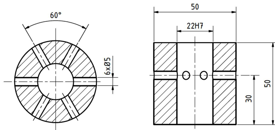
Obr. 1.1 Náčrt vyráběné součásti.
