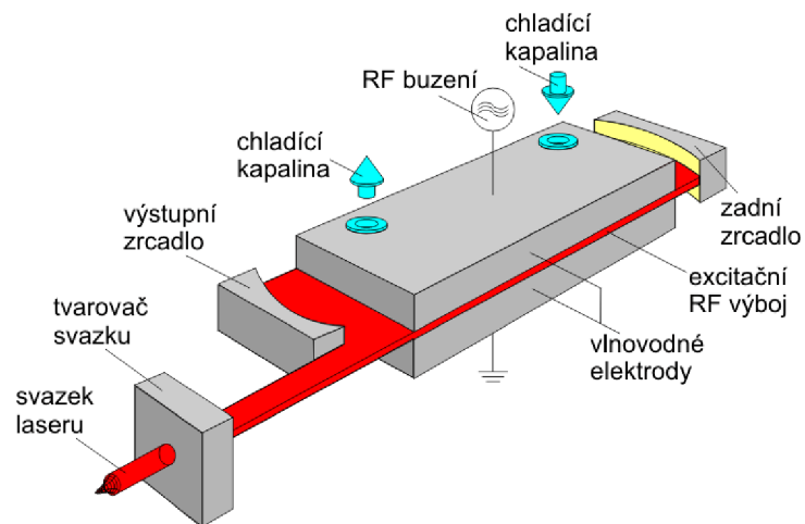
Obrázek 7 Radio-frekvenčně buzený slab \text{CO}_2 laser [10]
