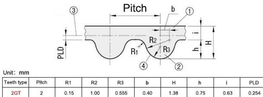
Obrázek 13 Technická data řemene GT2 [15]
