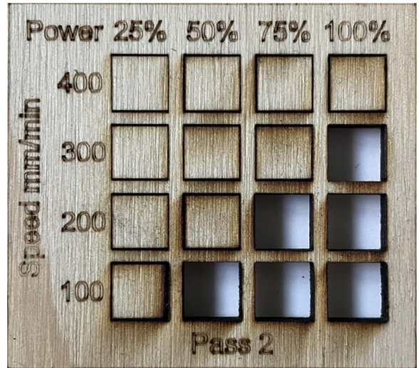
Obrázek 26 Dvě projetí řezu – borovicová překližka (4 mm)
