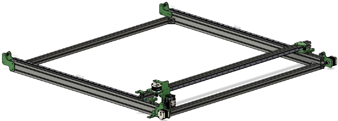
Obrázek 9 3D model gravírovacího zařízení v Autodesk Fusion 360
