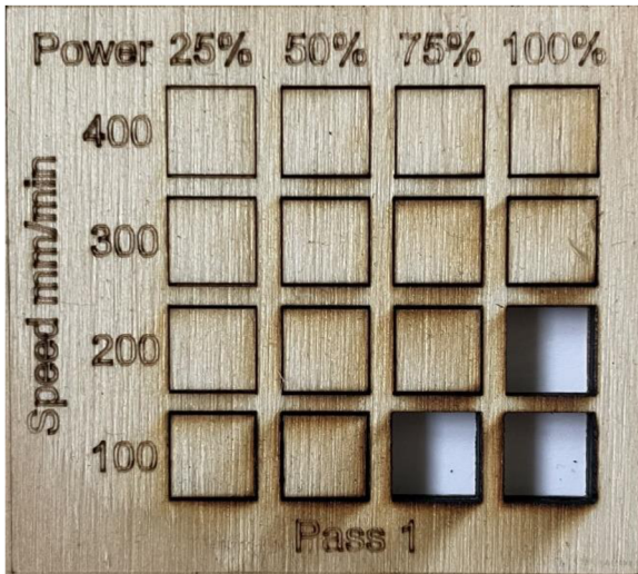
Obrázek 25 Jedno projetí řezu – borovicová překližka (4 mm)
