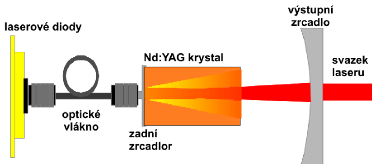
Obrázek 4 Nd:YAG laser se zadním buzením diodami [10]
