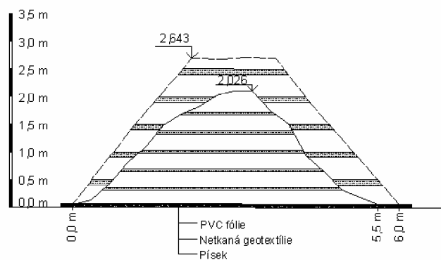
ŘEZ A-A' VE VZDÁLENOSTI 3 m
