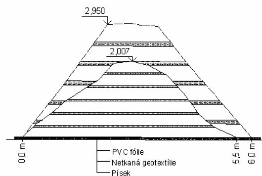
ŘEZ B-B' VE VZDÁLENOSTI 5 m
